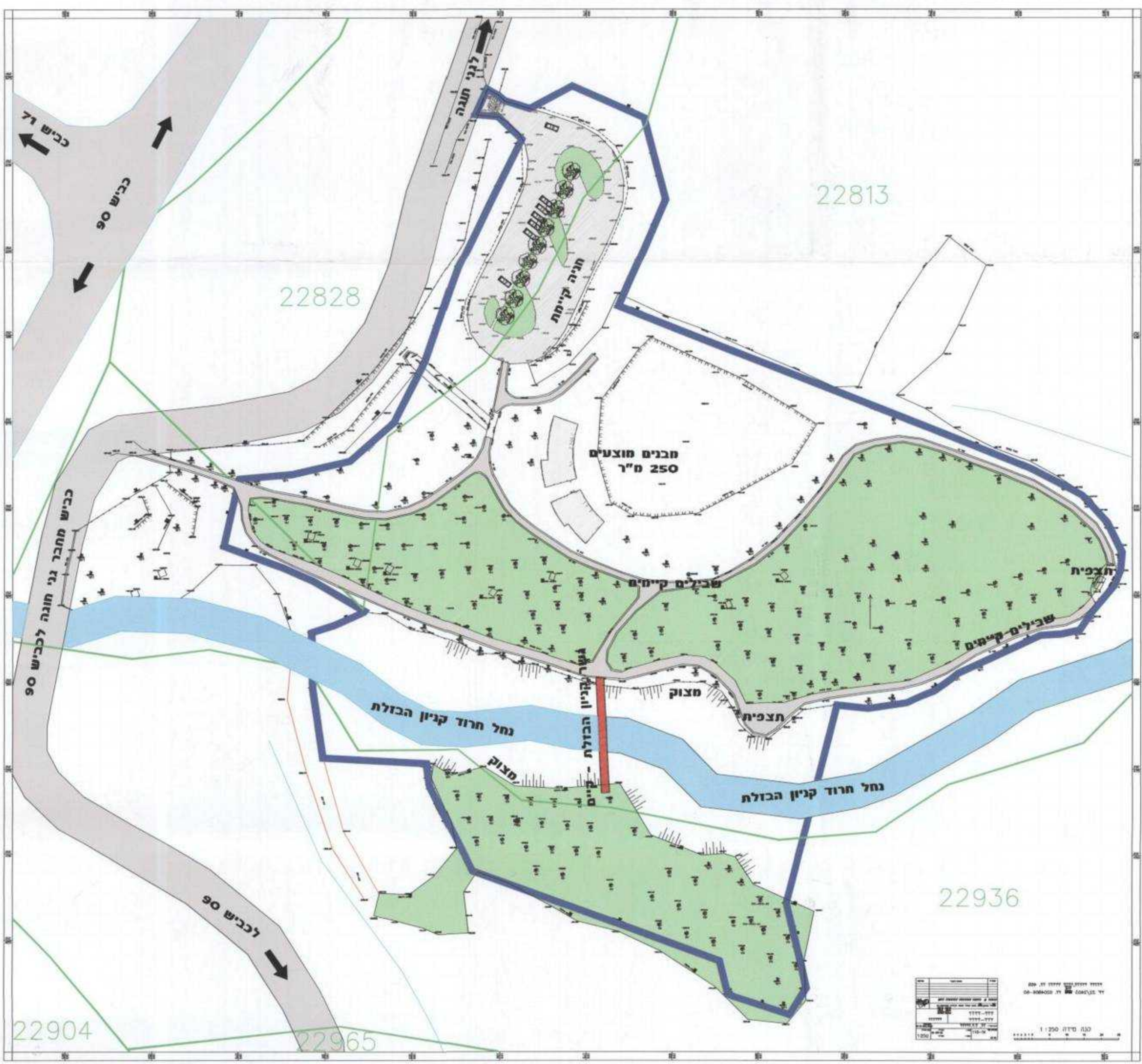
1:1250
