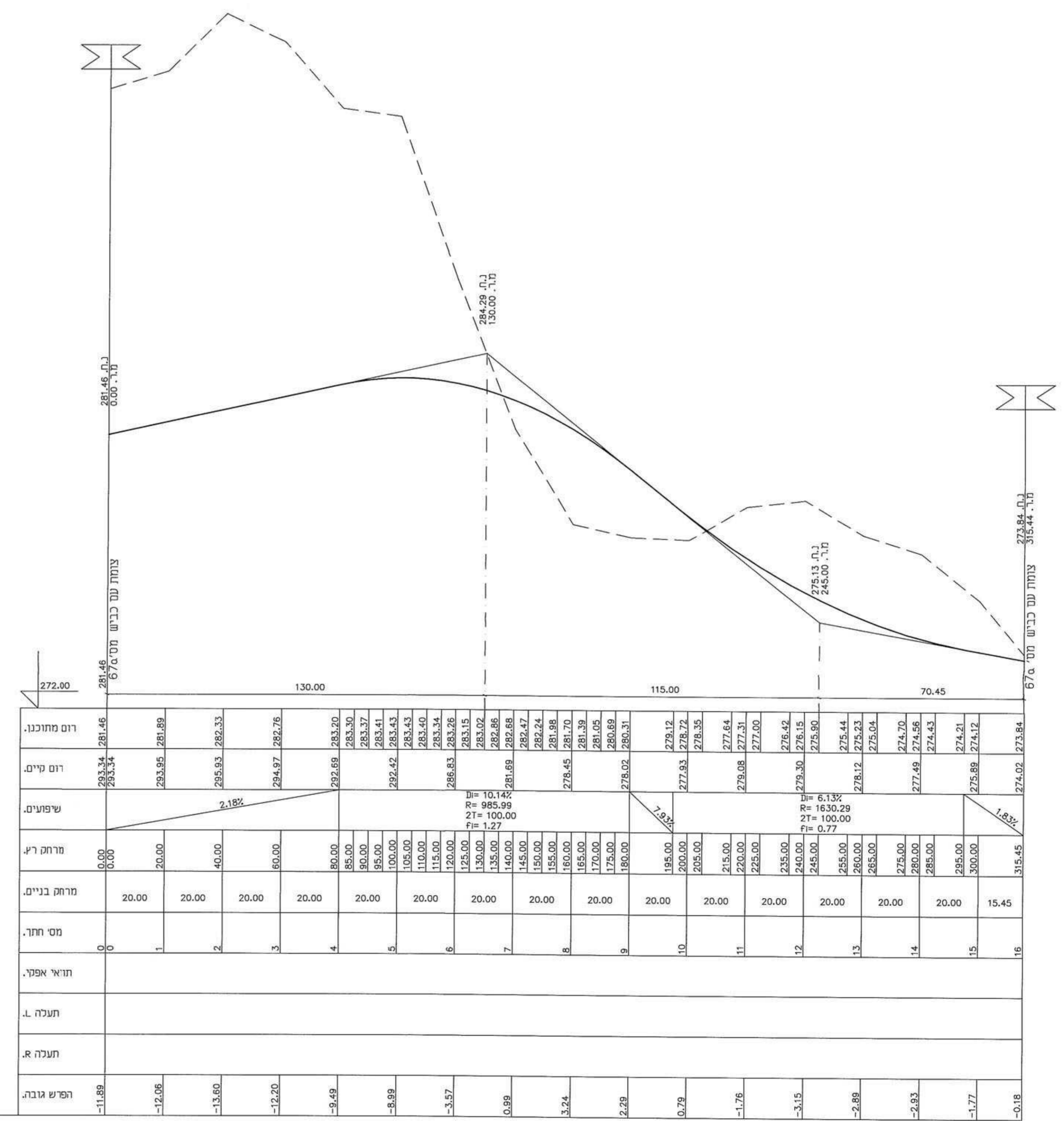
קנה מידה 1:100 / 1000
