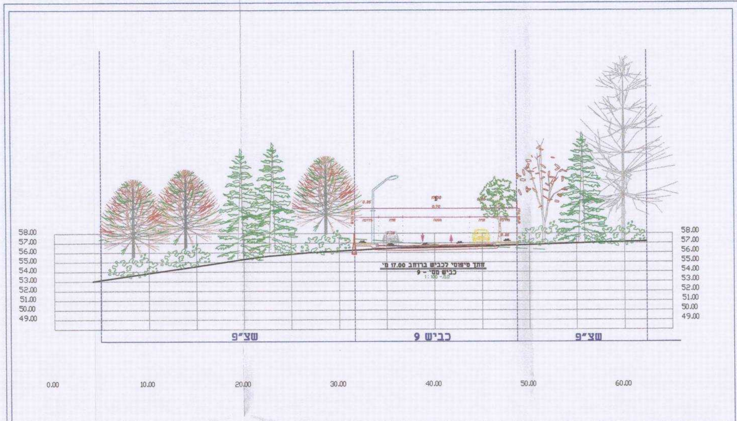
חתך 6-6
