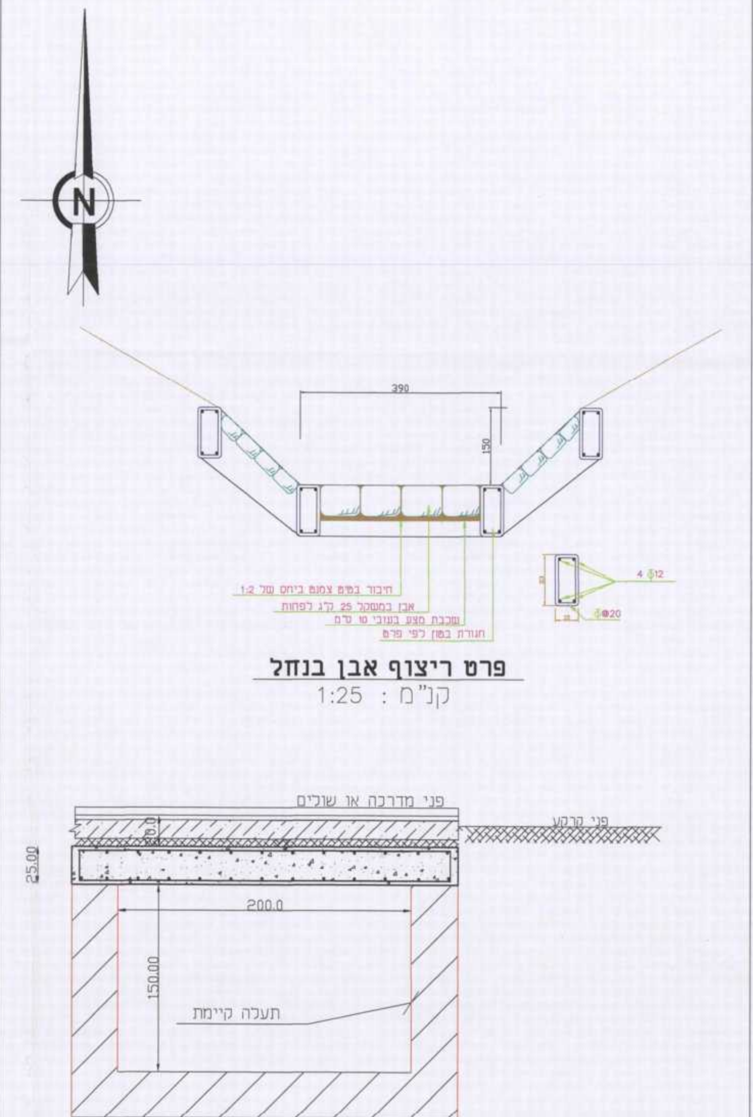
פרט תעלה תת קרקעי
