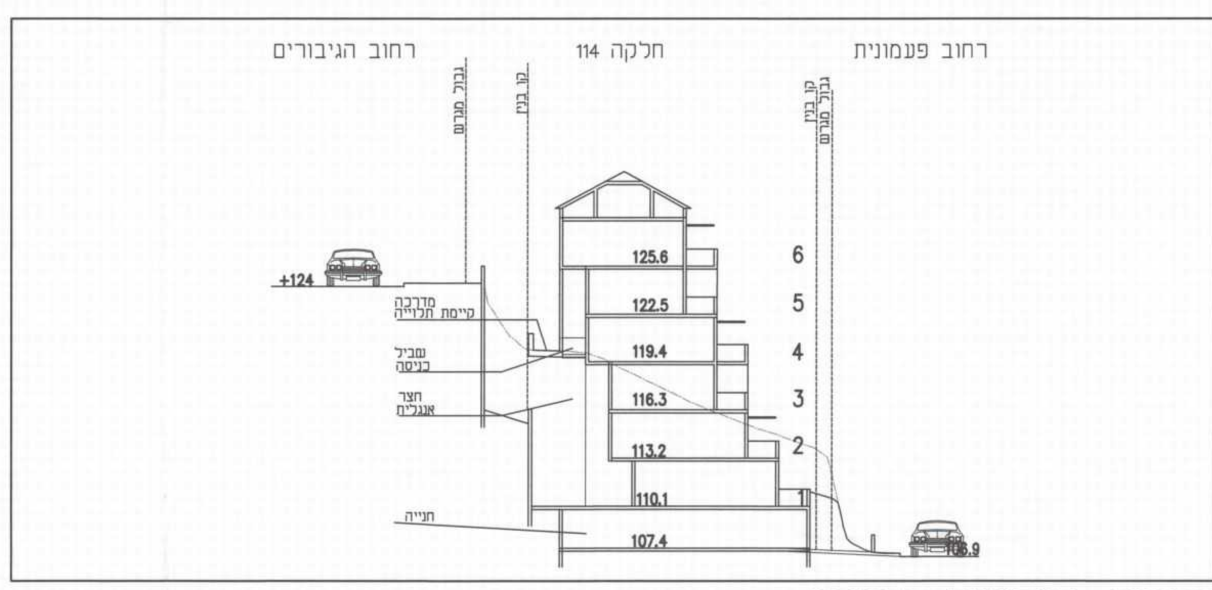
חתך תכנית בינוי
