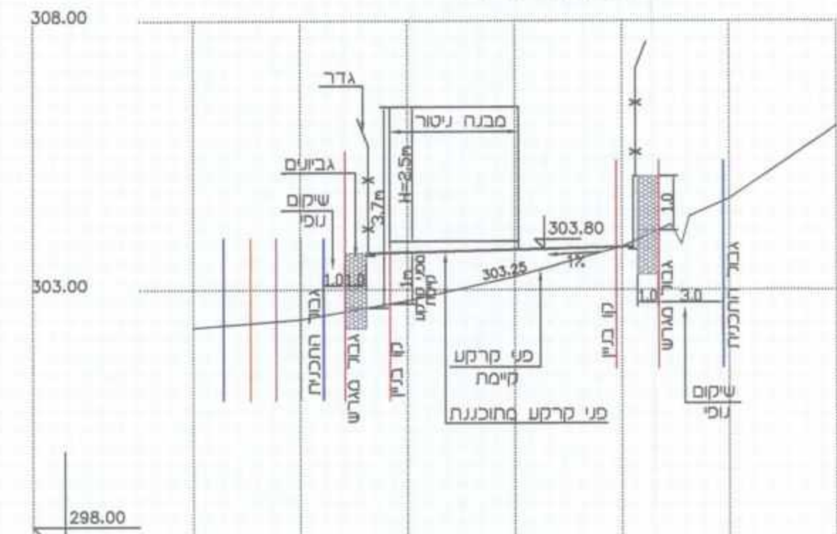
חזת א 1 : 100\250
