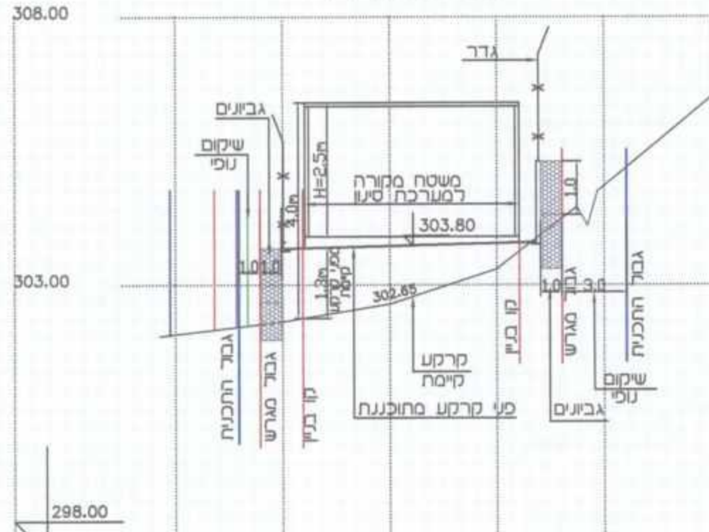
חזת ב 1 : 100\250
