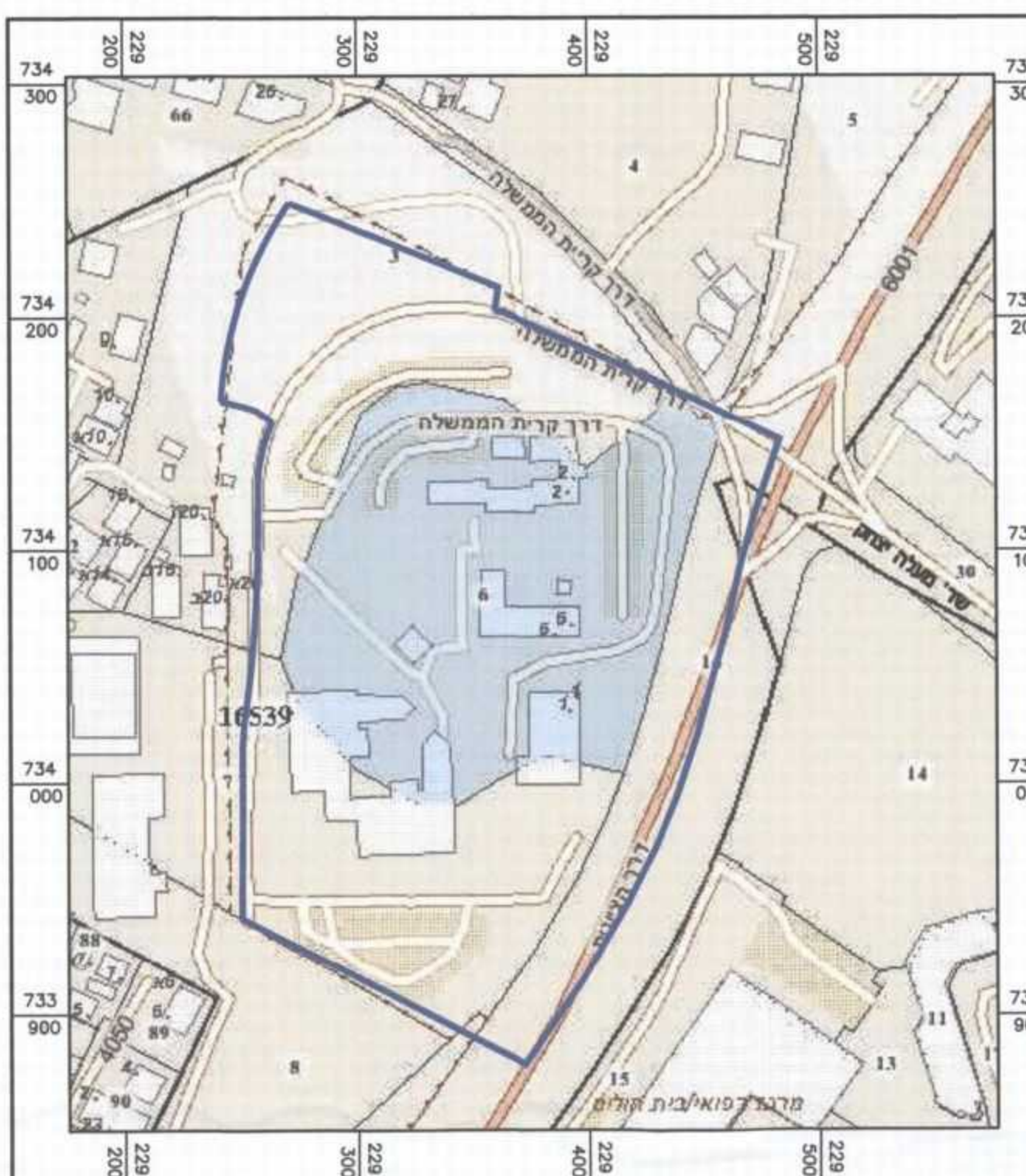
תרשים הסביבה 1:2500
