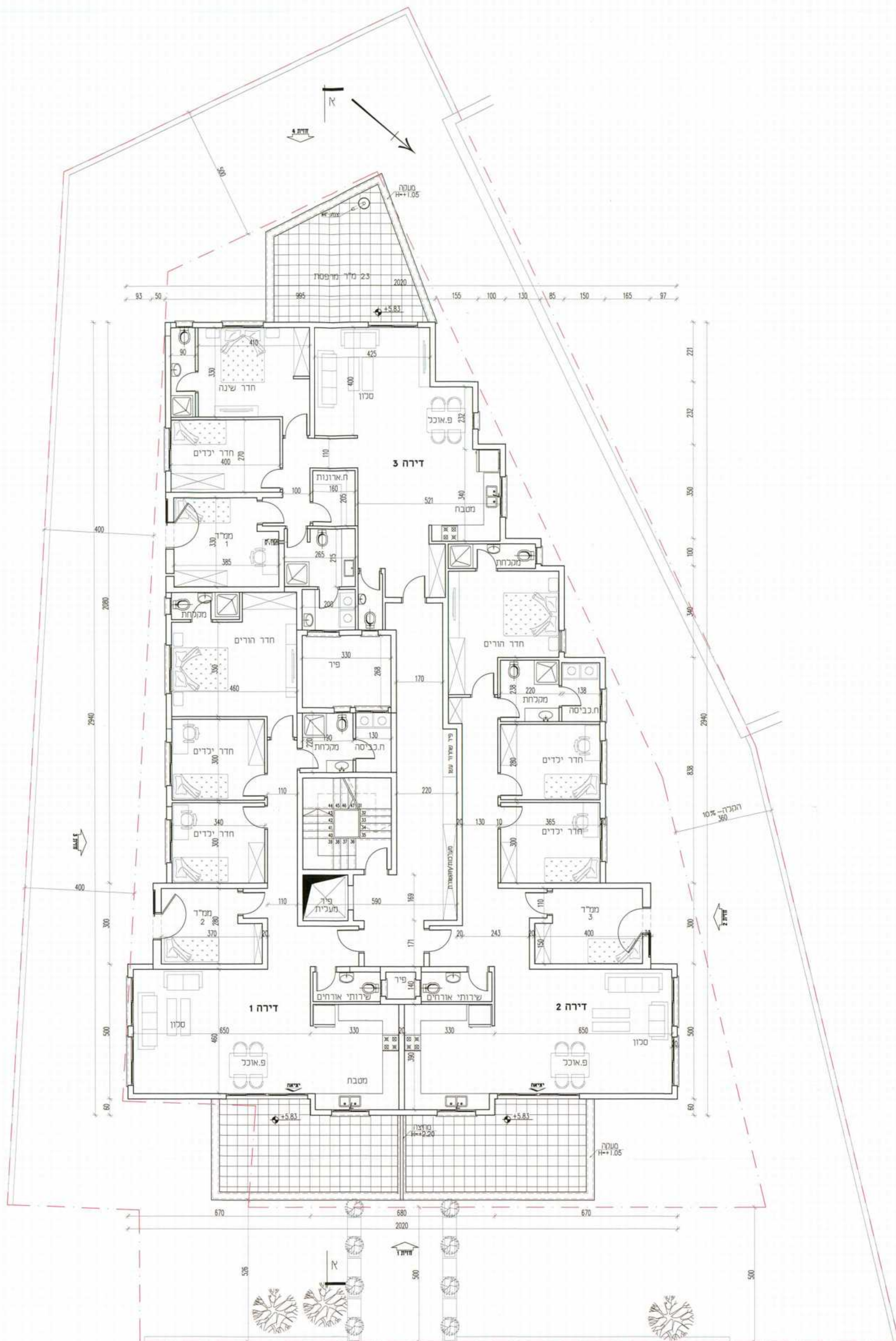
קומה טיפוסית גודל דירה לא עובר 120 מ"ר קנ"מ 1:100
