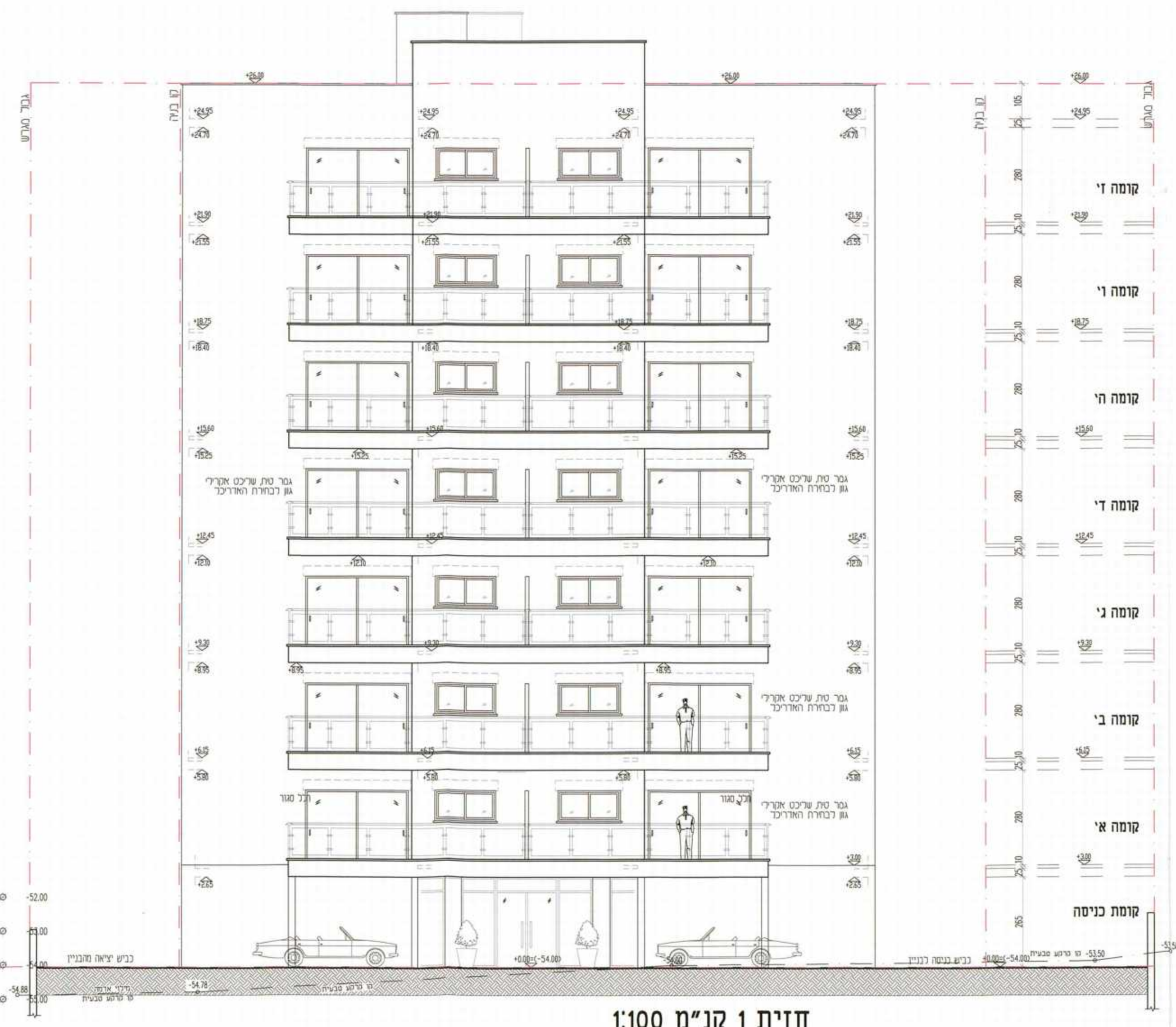
חזית 1 קנ"מ 1:100
