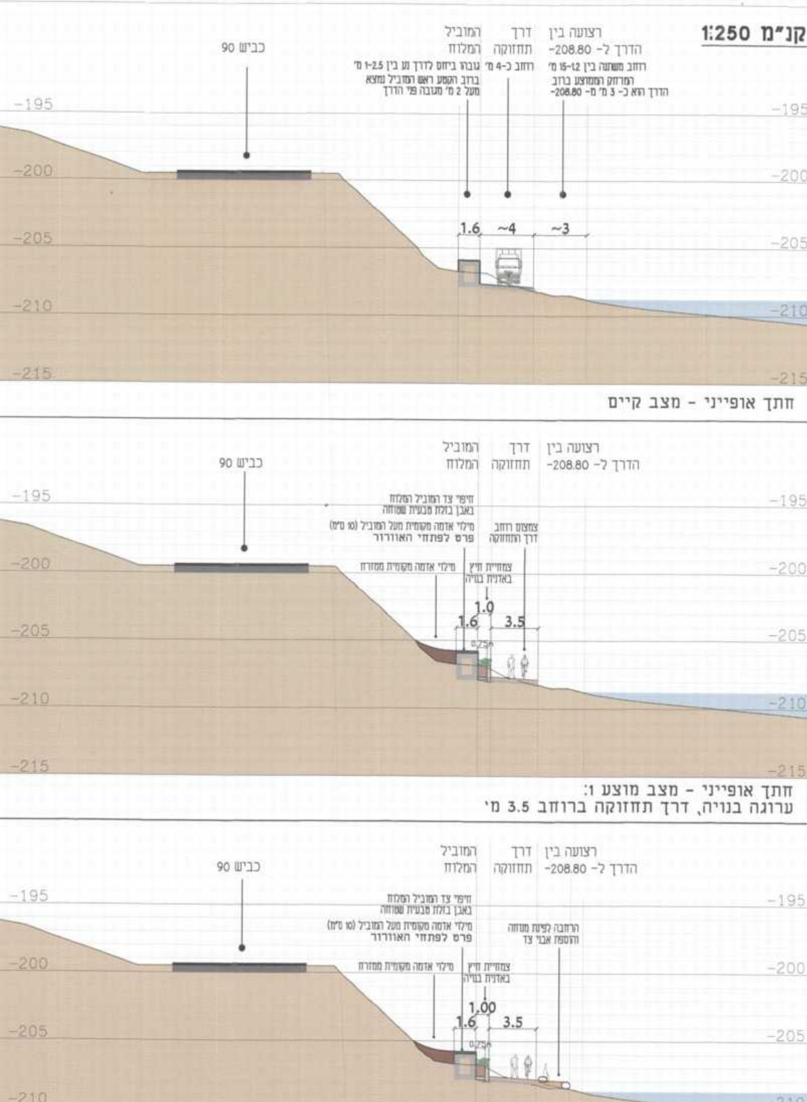
חתך אופייני - מצב מוצע 1: ערוגה בנויה, דרך תחזוקה ברוחב 3.5 מ' פינוט מנוחה (עד לגבול המצוק)
