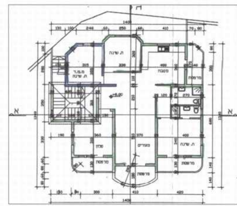
קומה ג' - מוצע
