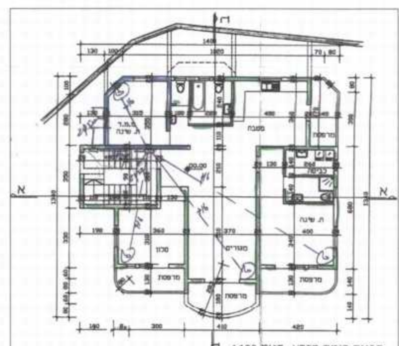
קומת קרקע - קיים
