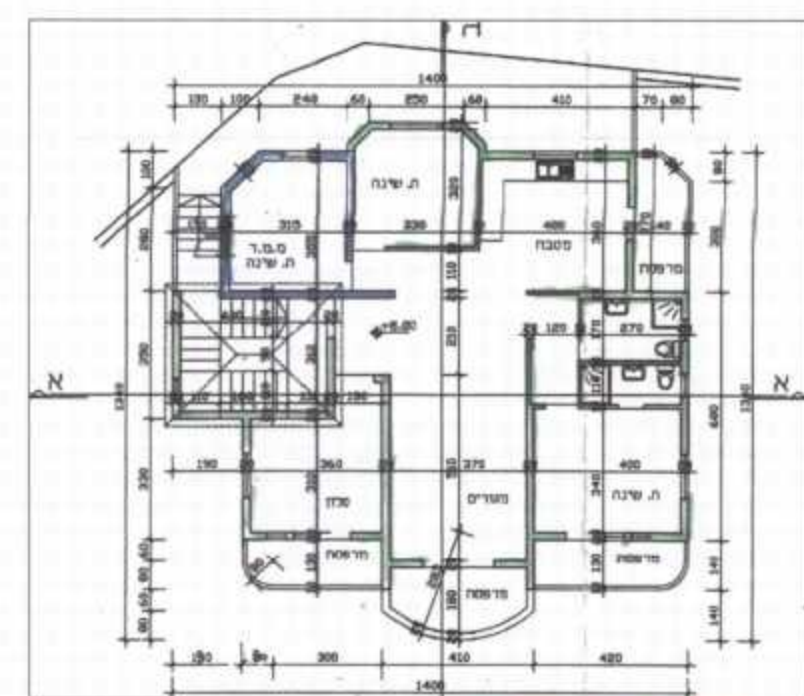
קומה ד' - מוצע
