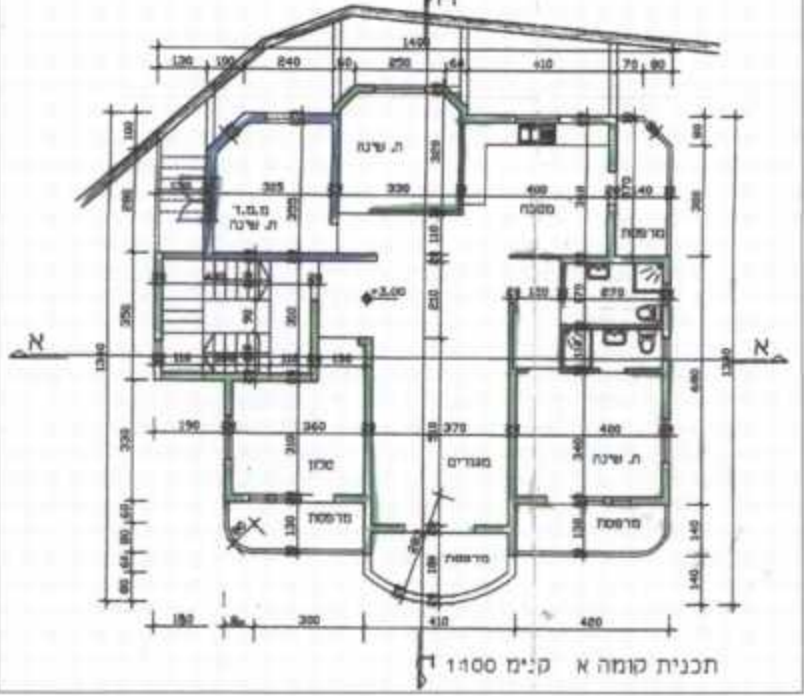
קומה א - קיים
