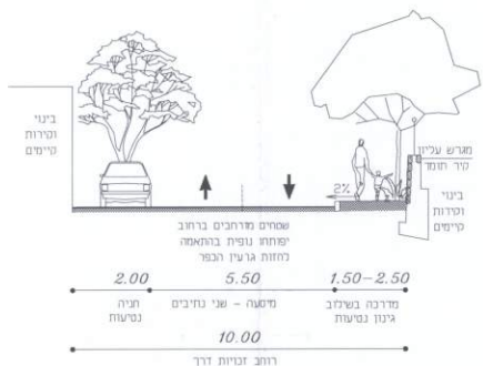
רחוב 10 מ' - טבעת גרעין הכפר-כבישים מדרכה-מסעה-מדרכה
