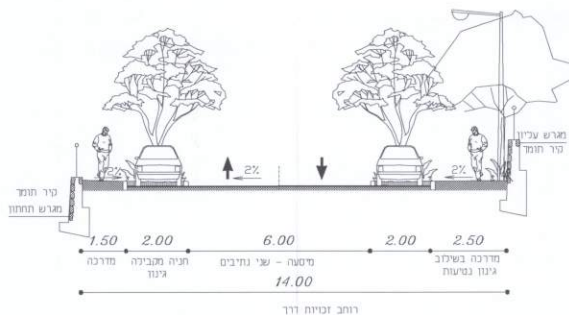
רחוב 14 מ' - חתך טיפוסי רחובות מוצעים מדרכה-חניה-מסעה-חניה-מדרכה
