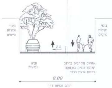
רחוב 10-8 מ' - סממאות וסבעת גרעין הכפר רחוב משולב
