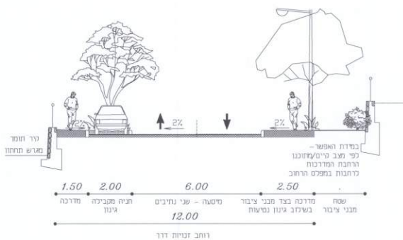
רחוב 12 מ' - חתך טיפוסי לאזור מבני ציבור מדרכה-מסעה-חניה-מדרכה
