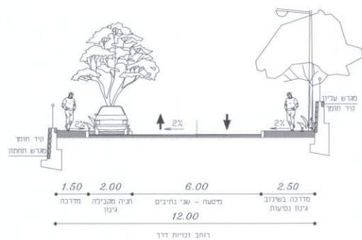
רחוב 12 מ' - חתך טיפוסי לאזור מגורים מדרכה-מסעה-חניה-מדרכה
