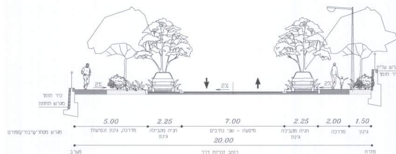
כביש כניסה ראשי - חתך רחוב 20 מ' גינן -מדרכה-חניה-מסעה-חניה-מדרכה-גינן
