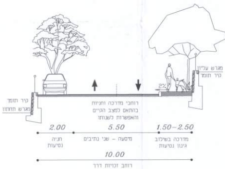
רחוב 10 מ' - חתך טיפוסי-שיקום רחובות קיימים מדרכה-מסעה-מדרכה
