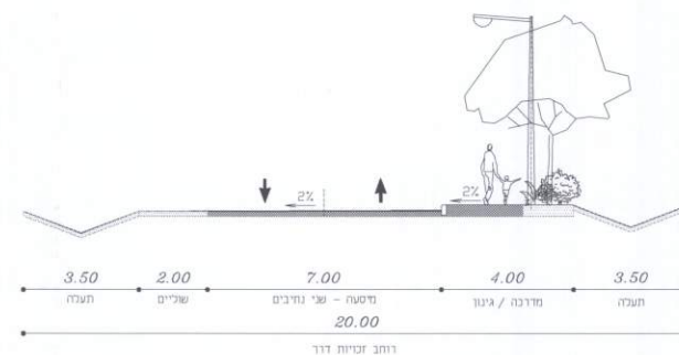
כביש גישה לאבירים - חתך רחוב 20 מ' תעלה-גינן /מדרכה-מסעה-שוליים-תעלה
