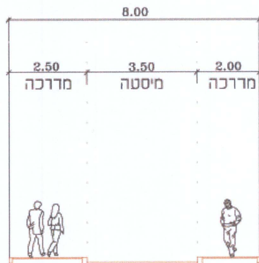
חותך טיפוסי - תחום דרך 10.00 מ' רחוב מס' 6 (בין חתכים 604-600) קנ"מ 100
