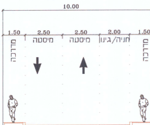
חותך טיפוסי - תחום דרך 10.00 מ' רחוב מס' 7 ת"מ סטוד
