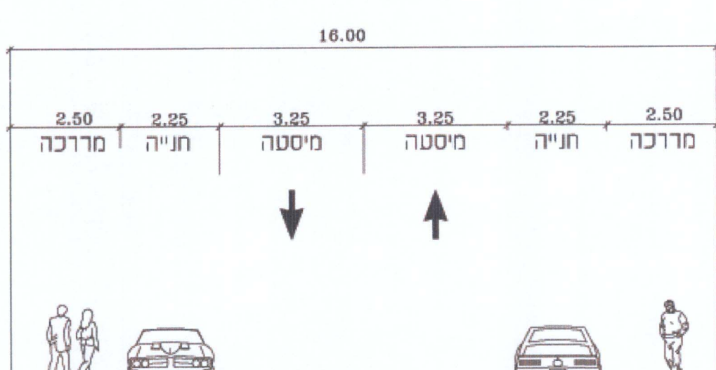
חוקך טיפוסי - תחום דרך 16.00 מ' רחוב מס' 80 קנ"מ 100
