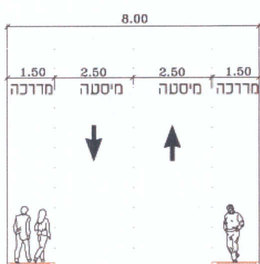
חתך טיפוסי - תחום דרך 8.00 מ' רחוב מס' 140 קט"מ 100
