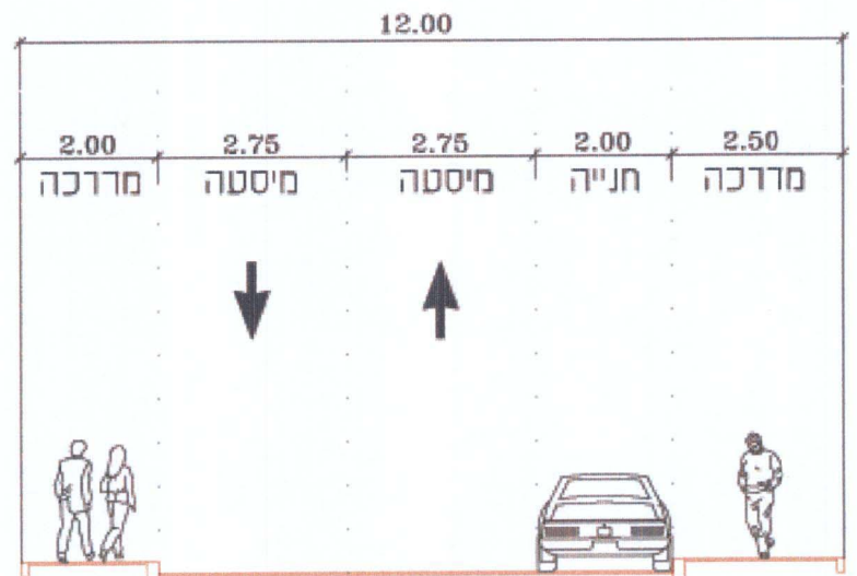
חוק טיפוסי - תחום דרך 12.00 מ' רחוב מס' 2 (בין חתכים 230-258) קט"מ 100
