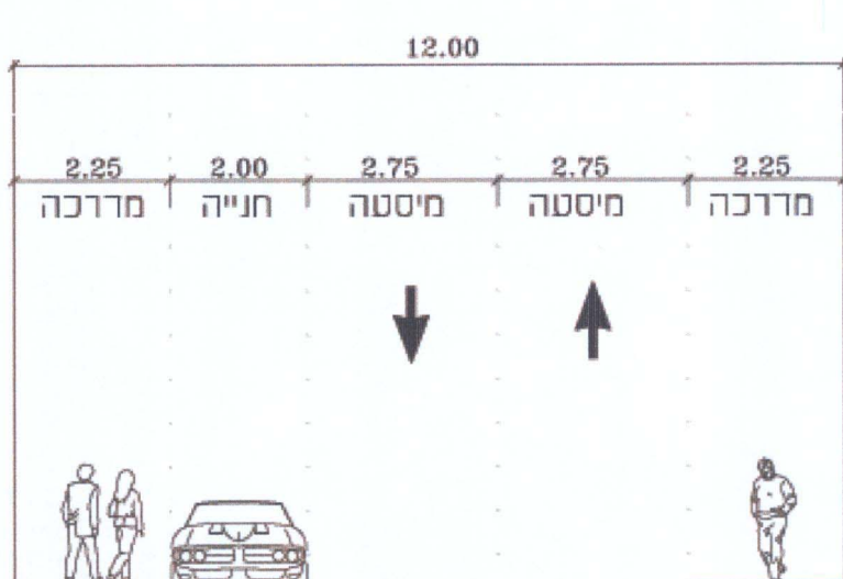
חתך טיפוסי - תחום דרך 12.00 מ' רחוב מס' 90 קו"מ 100
