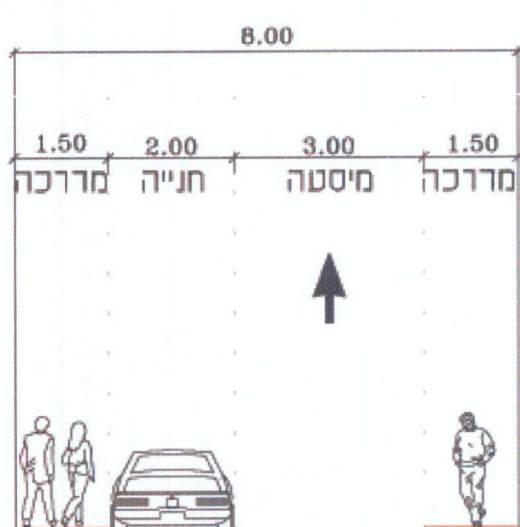
חתך טיפוסי - תחום דרך 8.00 מ' רחוב מס' 5 קו"מ 100
