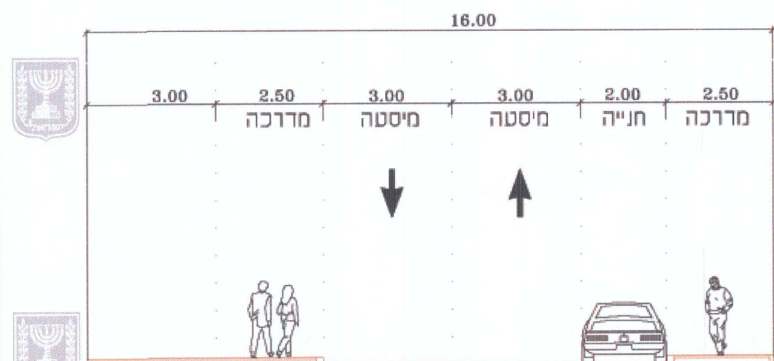
חתיך טיפוסי - תחום דרך 16.00 מ' רחוב מס' 4 (בין חתכים 145-232)
