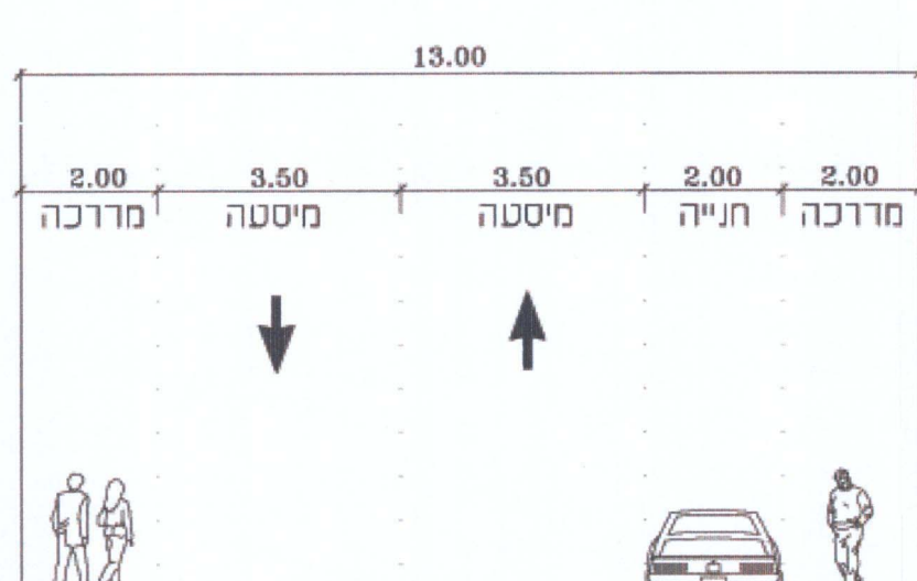
חנות טיפוסי - תחום דרך 13.00 מ' רחוב מס' 1 קמ"מ 100
