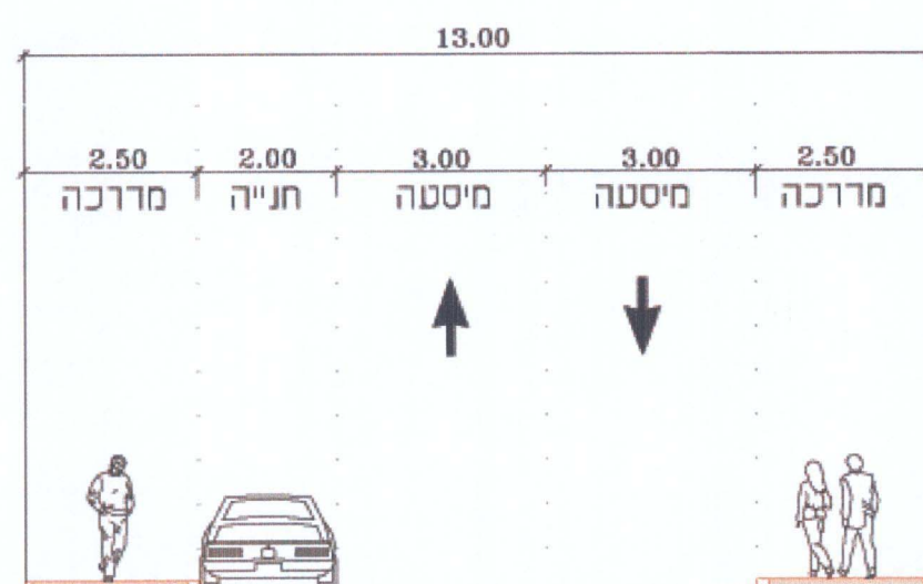
חוקר טיפוסי - תחום דרך 13.00 מ' רחוב מס' 10 (בין חתכים 145-232) קנ"מ 100
