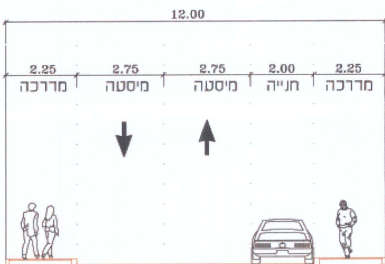
חותך טיפוסי - תחום דרך 12.00 מ' רחוב מס' 30 קו"מ 100
