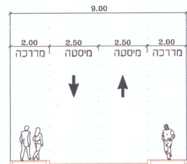
חתיך טיפוסי - תחום דרך 10.00 מ' רחוב מס' 2 (בין חתכים 220-230) קו"מ 100
