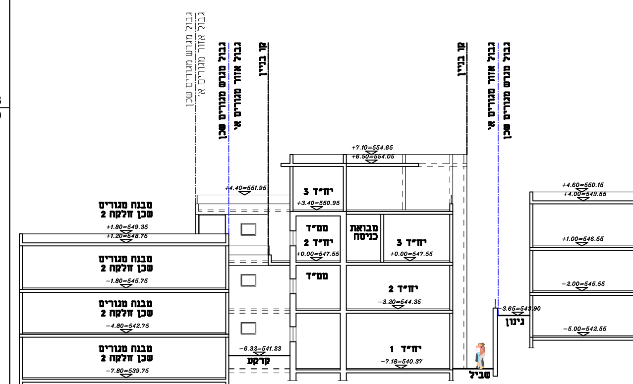
חתך ג-ג קנ"מ 1:250
