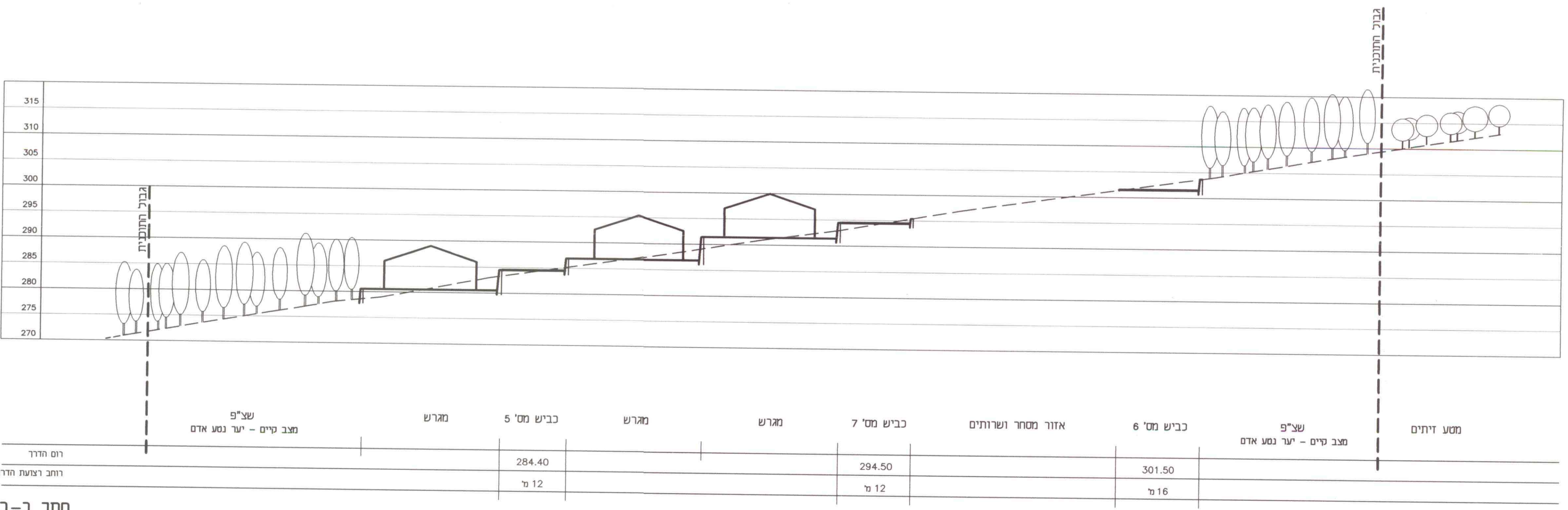
חתך ב-ב
