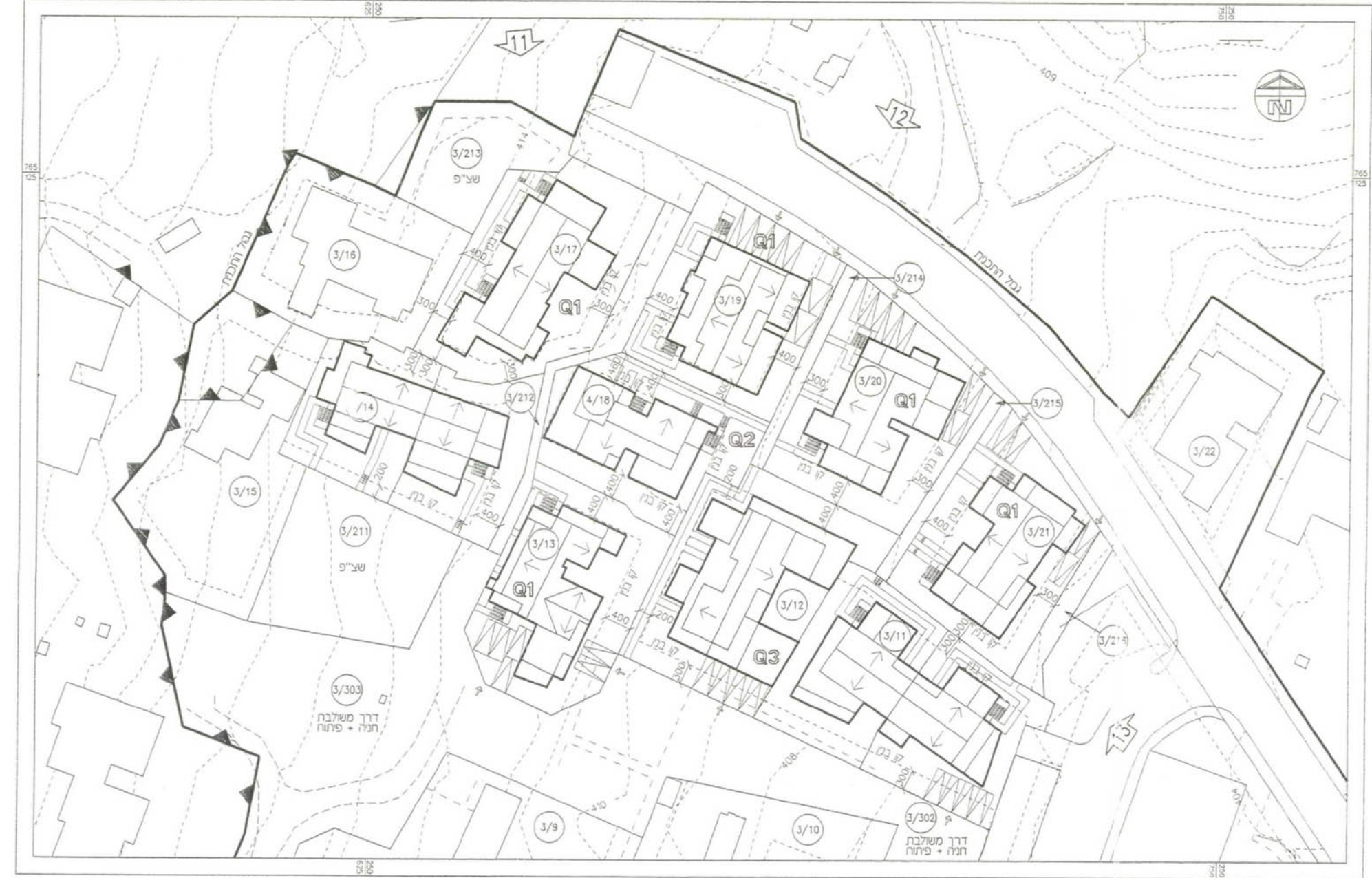
תכנית הדגמת בניו מקטע 'א' ק.מ. 1:500
