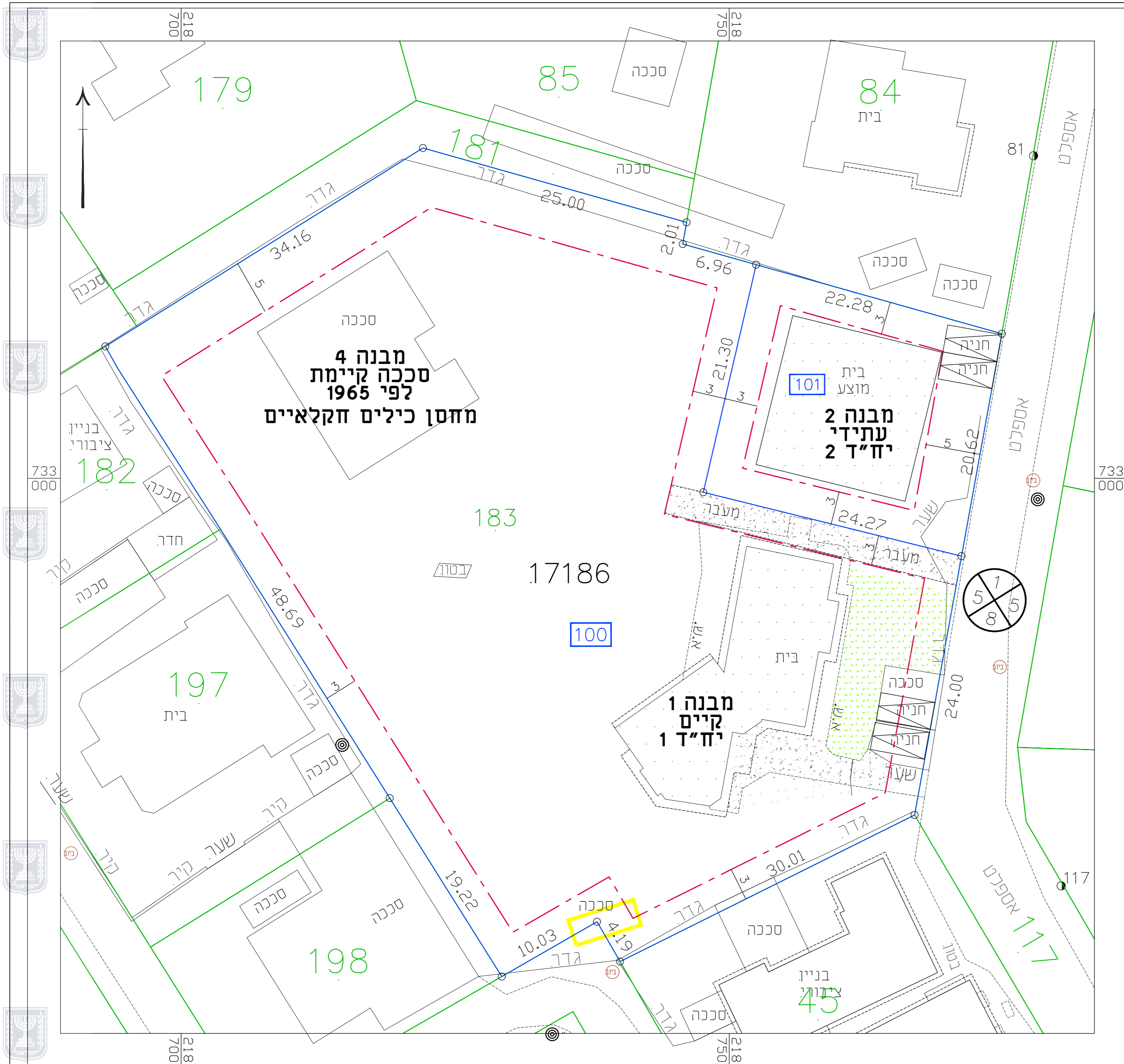
נספח בינוי קני"מ 1:250
