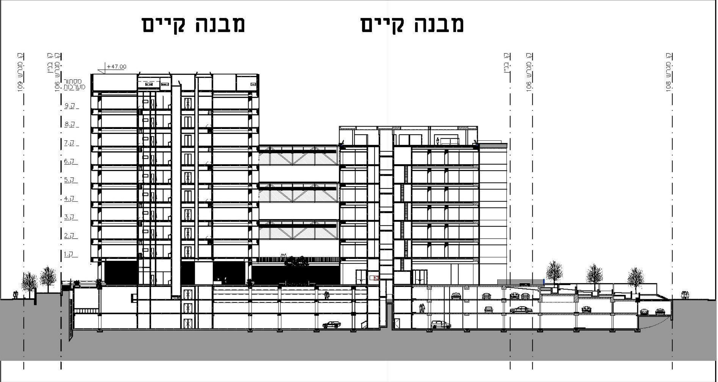
קנ"מ 1:1000 תכנית בינוי חתך 2-2
