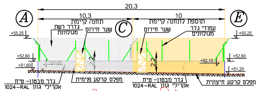
מבט F-B 1:200
