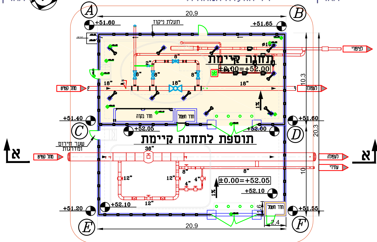
תכנית תחנת מגופים - כפר ברוך 1:200
