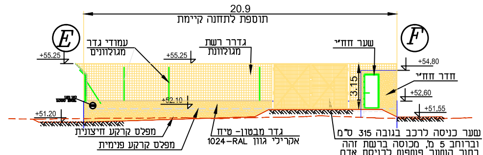
מבט F-E 1:200
