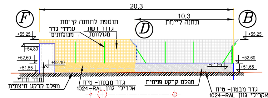
מבט F-B 1:200
