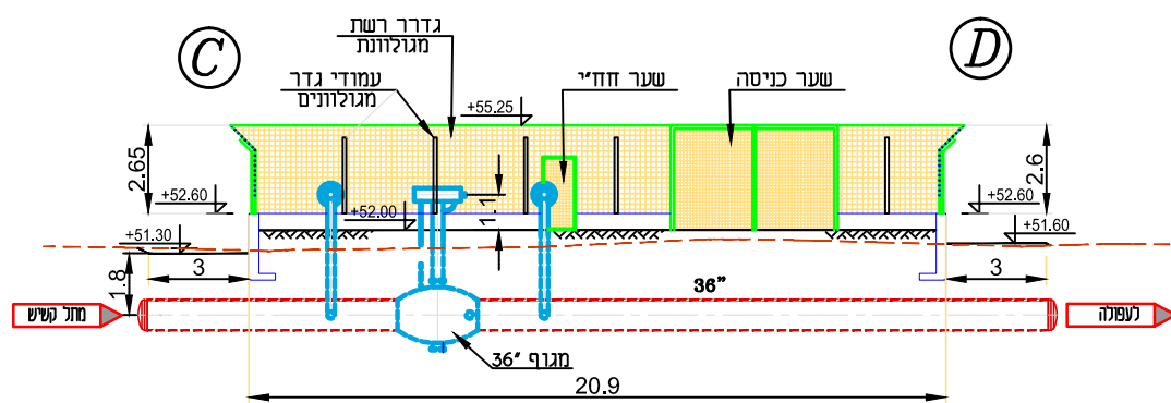
חתך א-א
