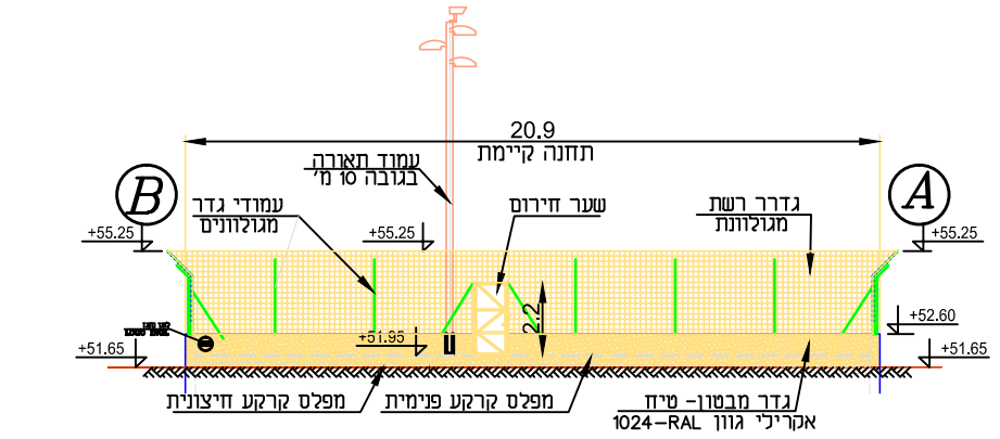
מבט A-B 1:200
