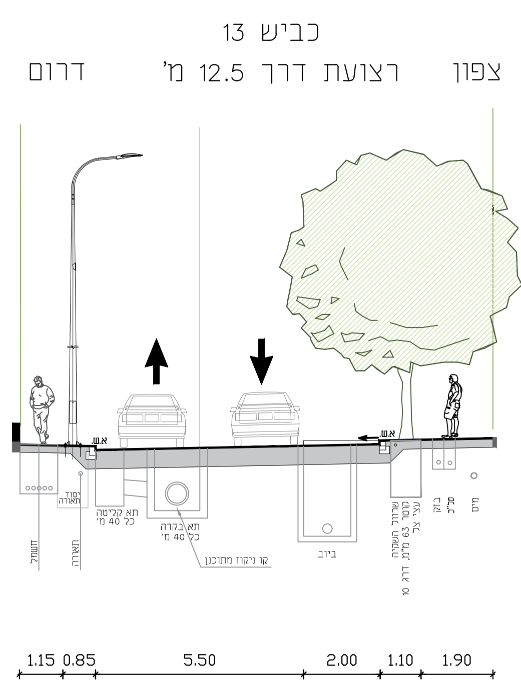
חזתי רחוב טיפוסיים 1:100
