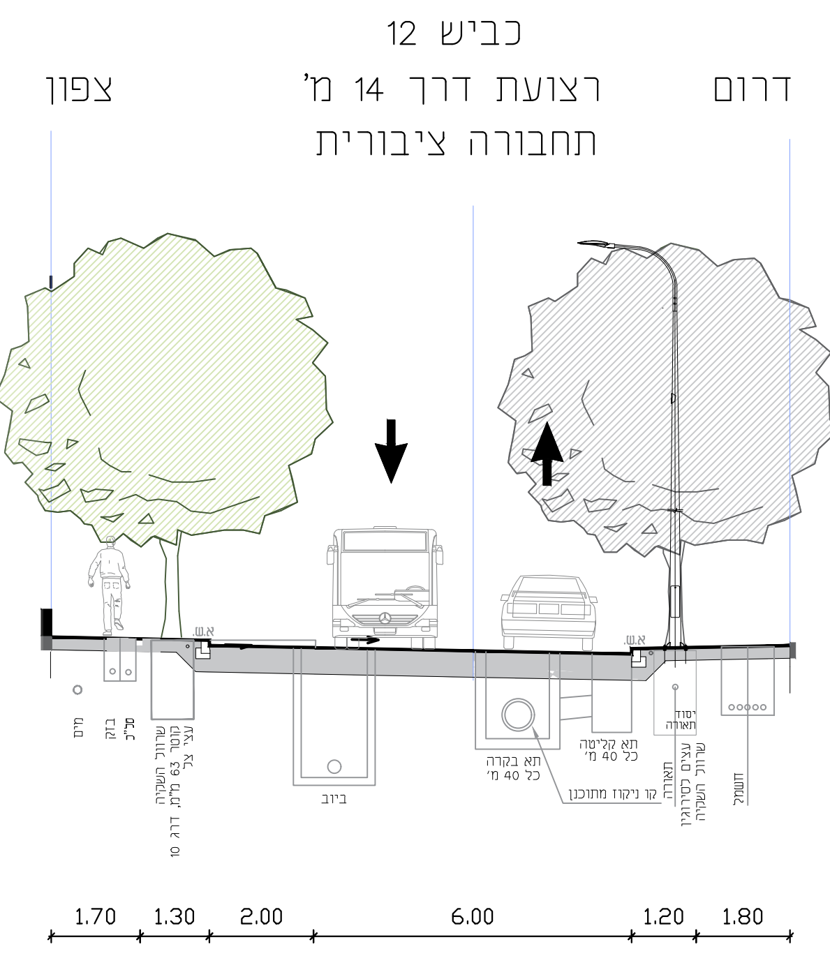
חזתי רחוב טיפוסיים 1:100
