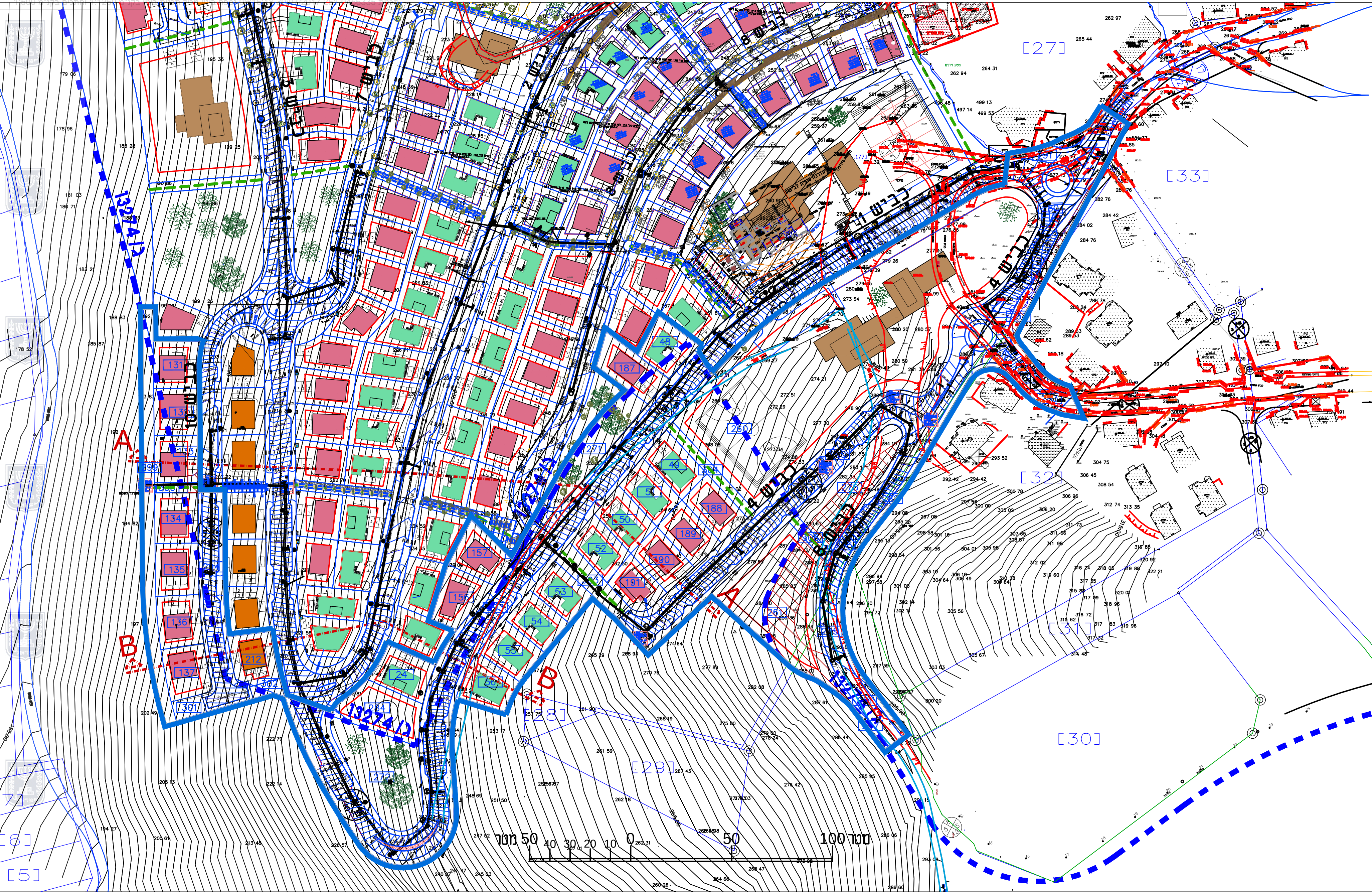
תכנית בנין קנ"ח 1:1250
