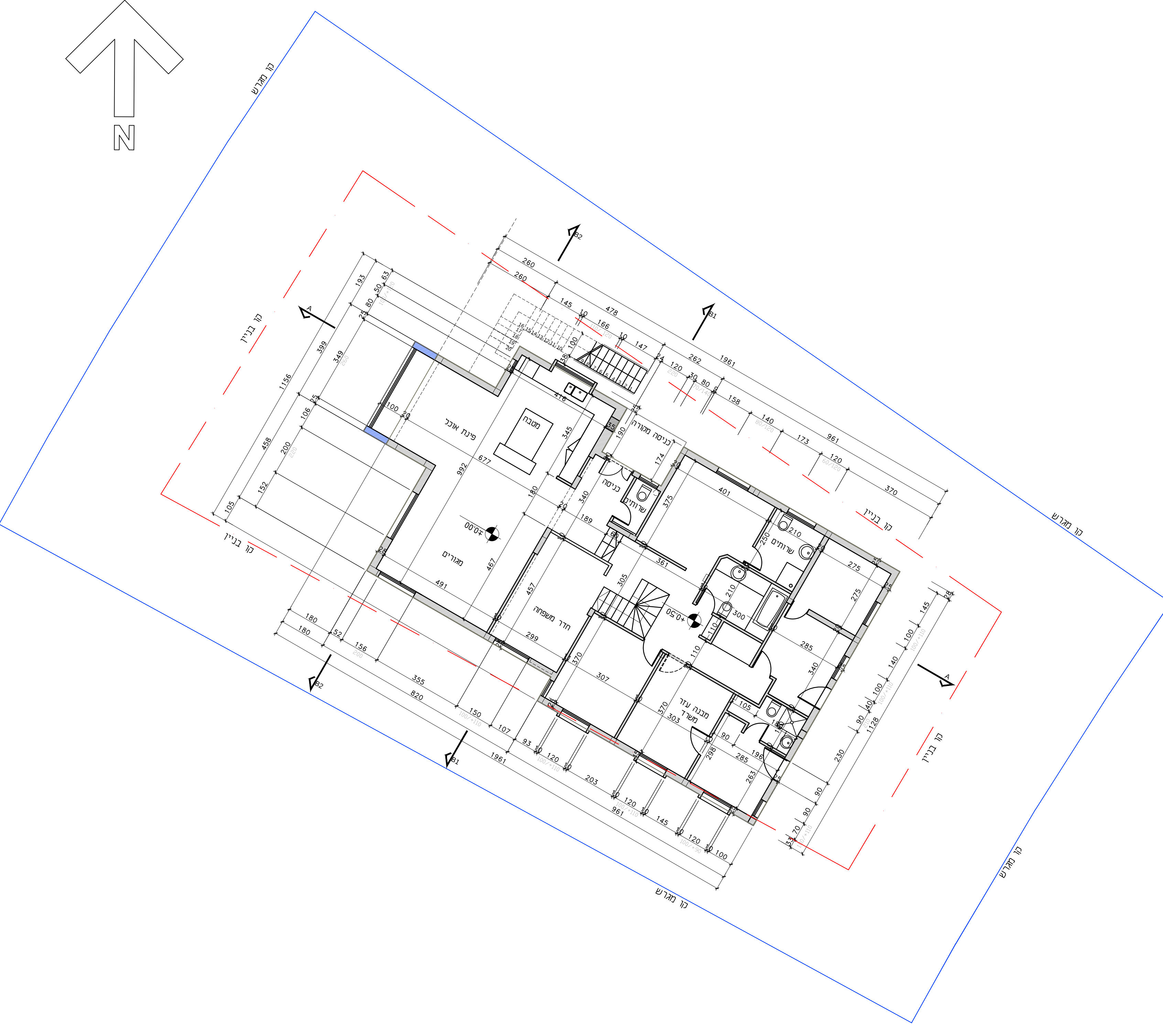
תכנית קומת קרקע 1:100
