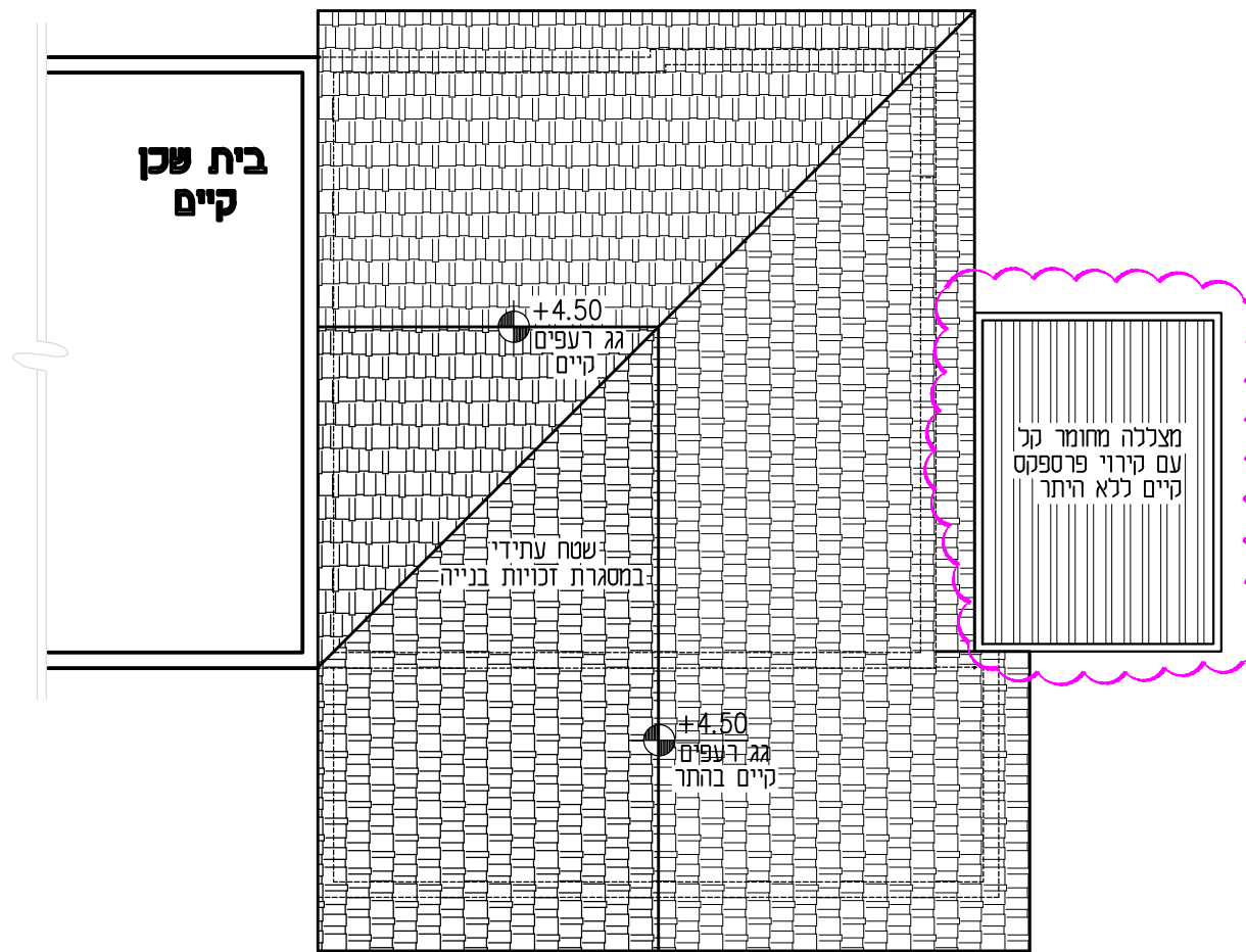
תכנית גגות 1 : 100
