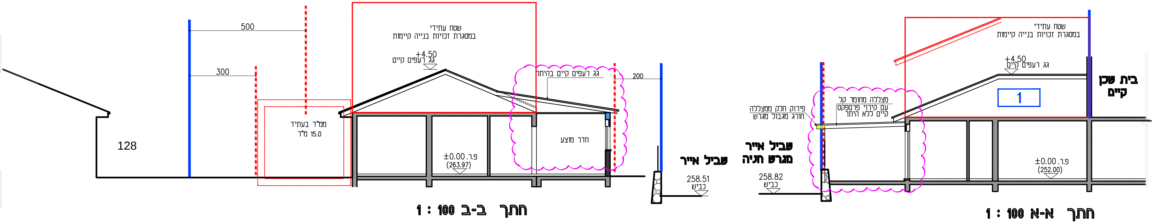
חתך א-א 1 : 100
