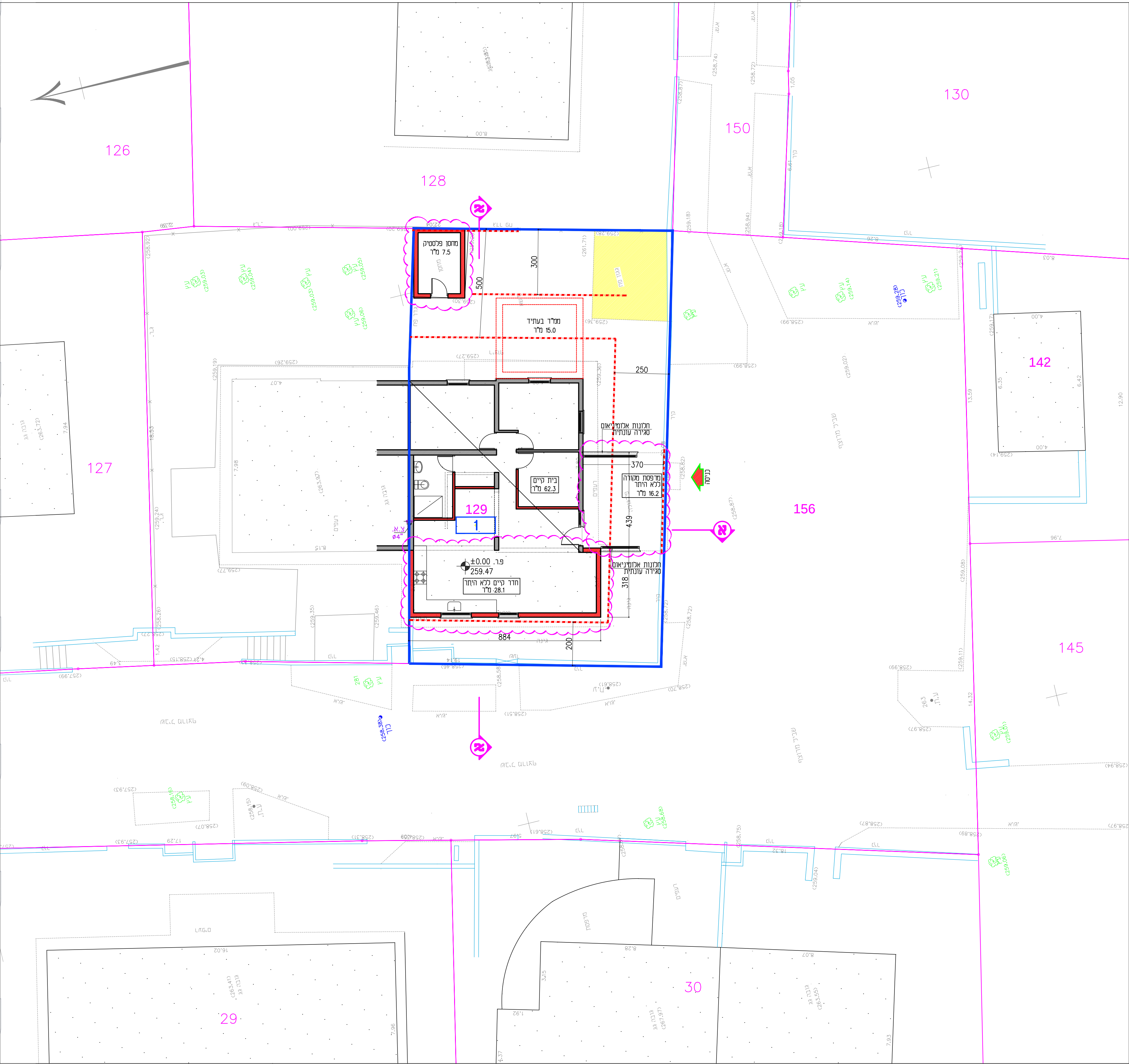
תכנית קומת כניסה 1 : 100
