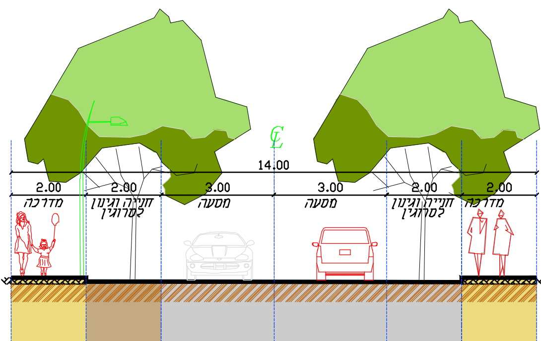
חוק ספוט לכביש 14 מ' כביש דו-סטרי עם חניה כפולה בשילוב גינון
