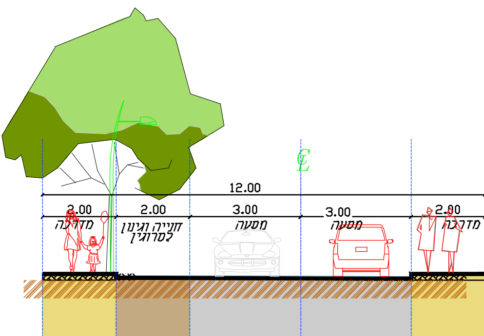
חוק ספוט לכביש 12 מ' כביש דו-סטרי
