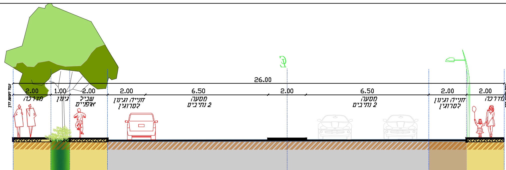
חוק ספוט לכביש 26 מ' כביש דו-סטרי עם סיינת נופית ושביל אופיים
