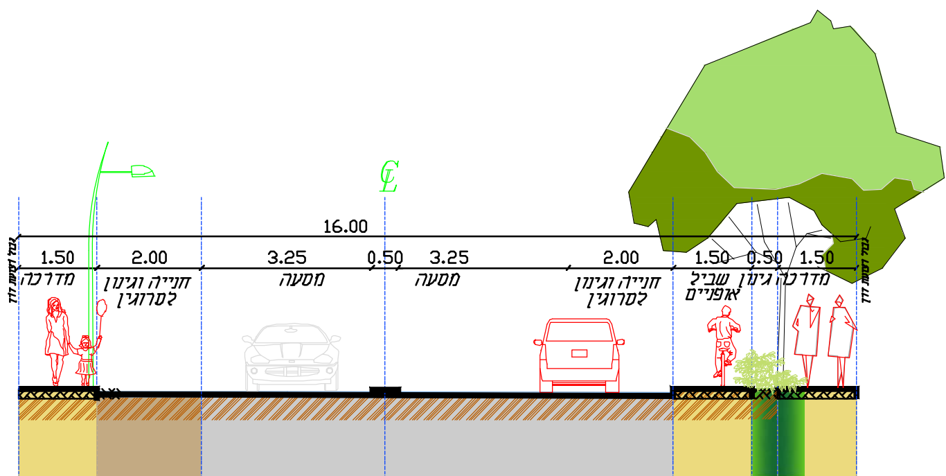
חוק ספוט לכביש 16 מ' כביש דו-סטרי עם סיינת נופית ושביל אופיים
