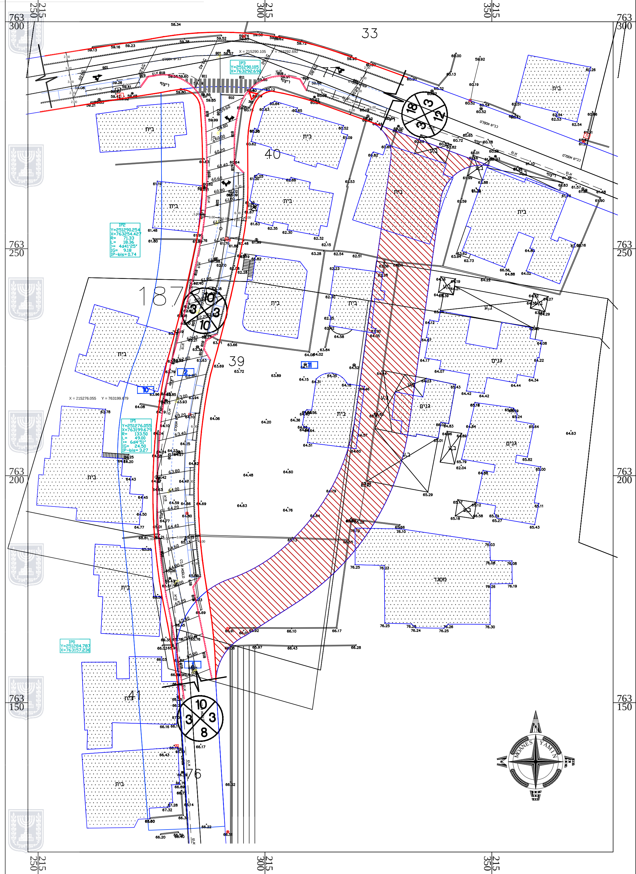
תכנית תנועה קני"מ 1 : 500
