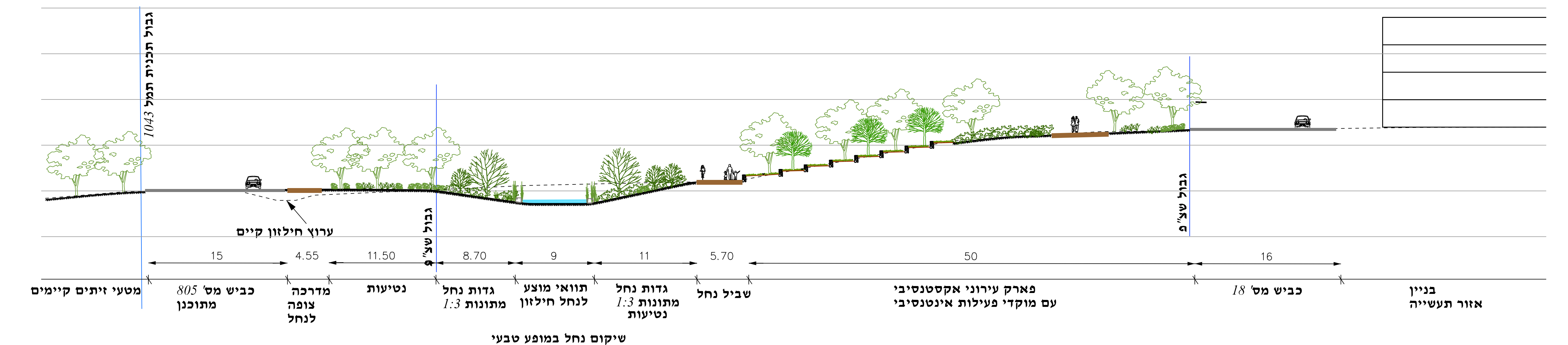
חתך ג-ג חתך נחל מלא עם דופן בינוי קנ"מ 1:250
