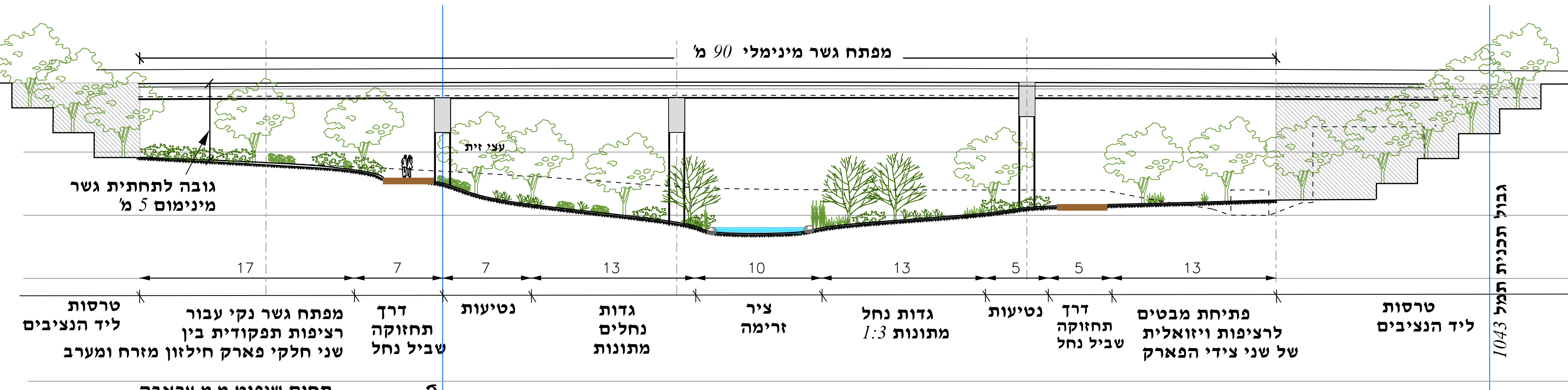
חתך ב-ב חציית כביש 804 מעל נחל חילזון קנ"מ 1:250 חזית מערבית - מצב מוצע
