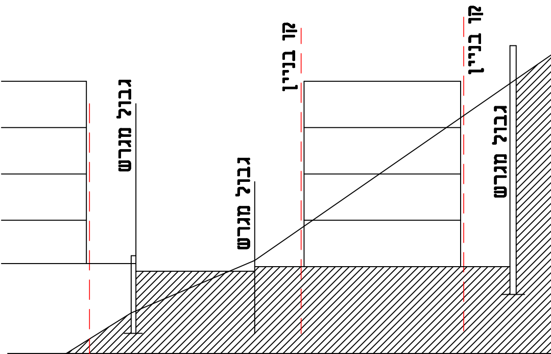
חתך סימתי למגרש 100\3
