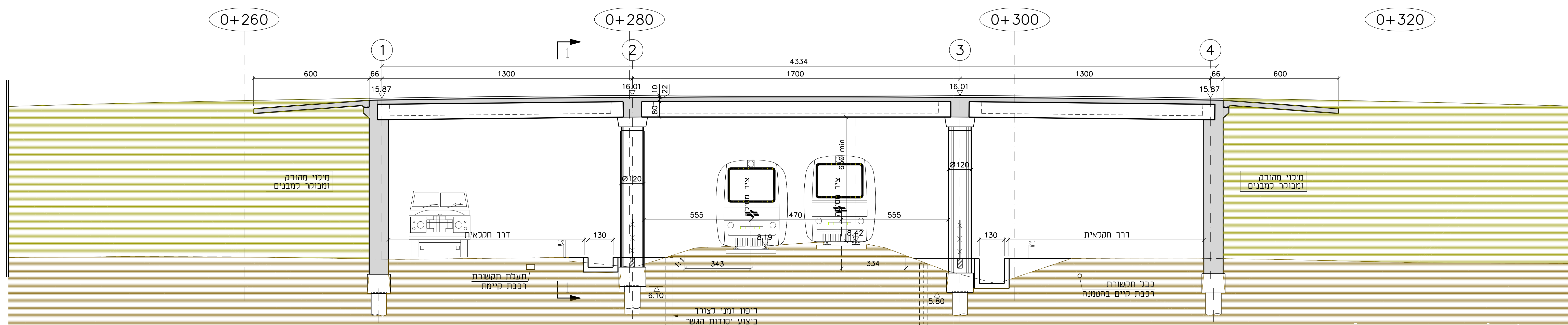
חתך לאורך בציר הגשר קנ"מ 1:100
