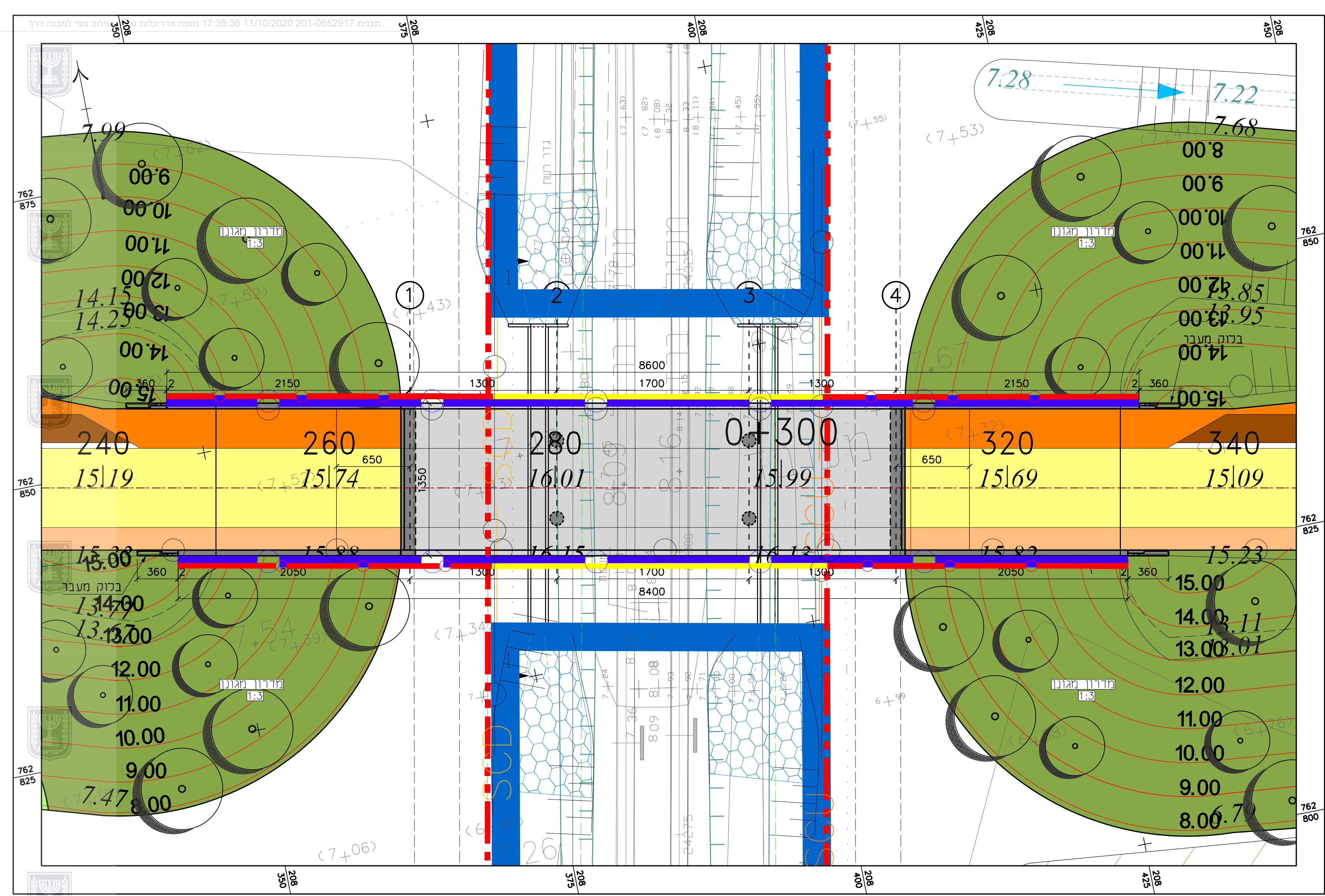
תווחה קנ"מ 1:250
