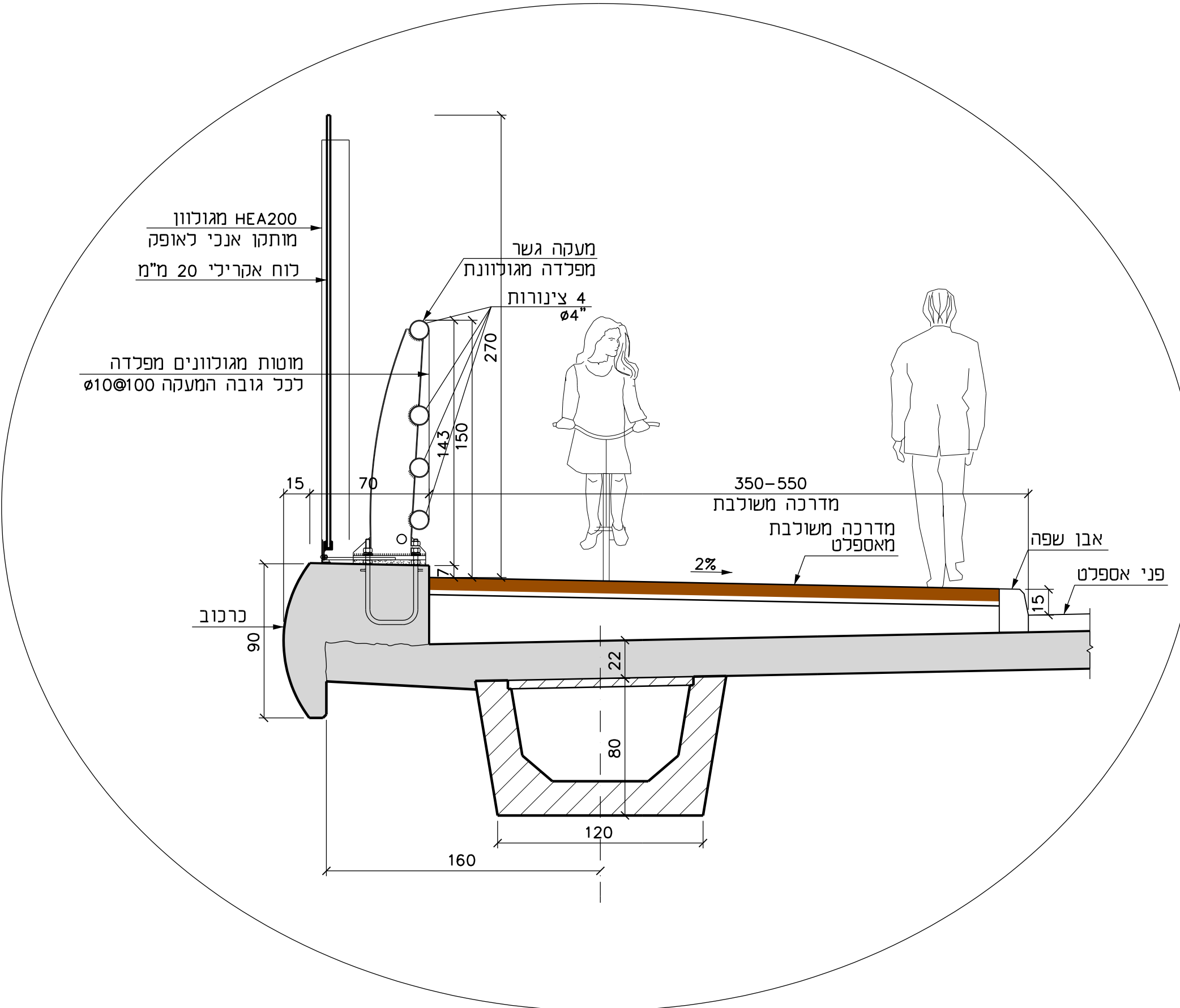
פרט A קנ"מ 1:25
