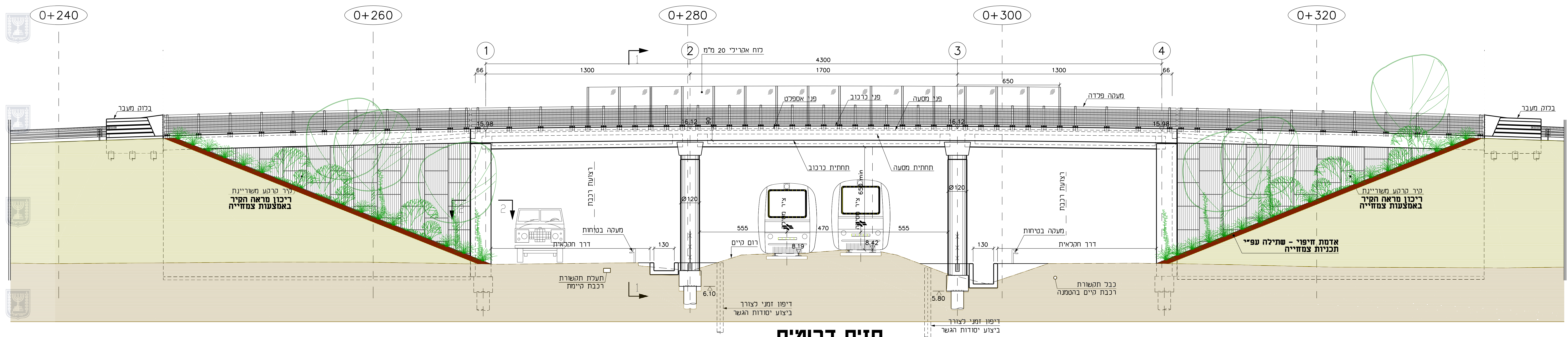
חזית דרומית קנ"מ 1:100
