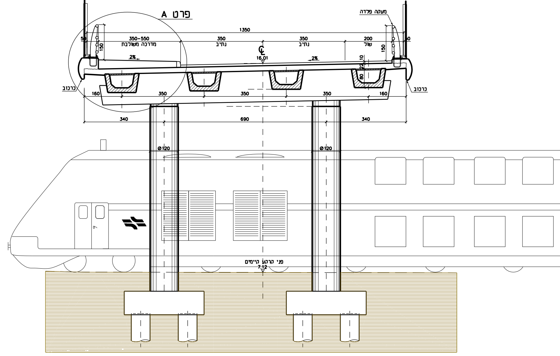
חתך 1-1 קנ"מ 1:100
