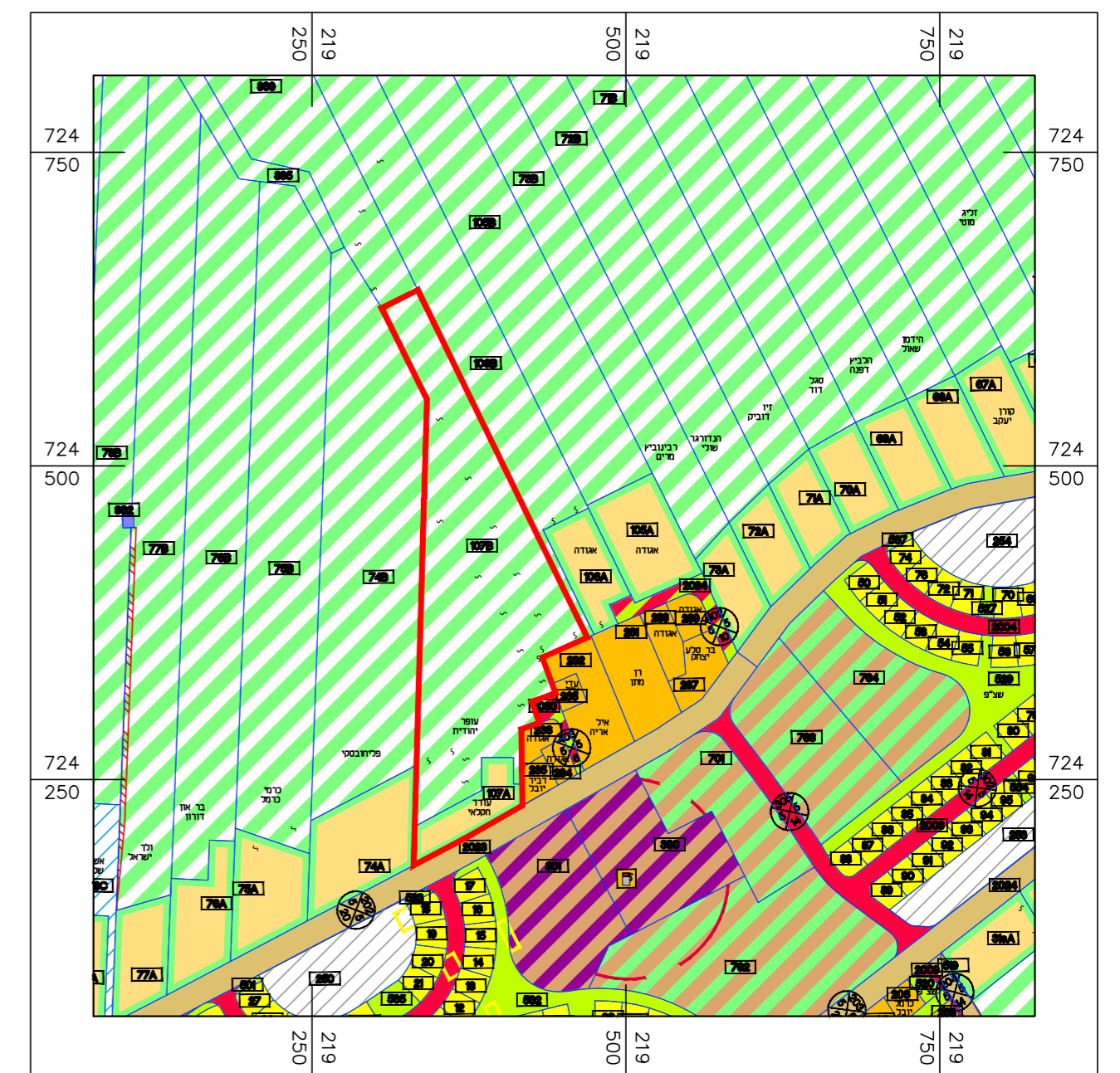
תרשים סביבה 1:5000
