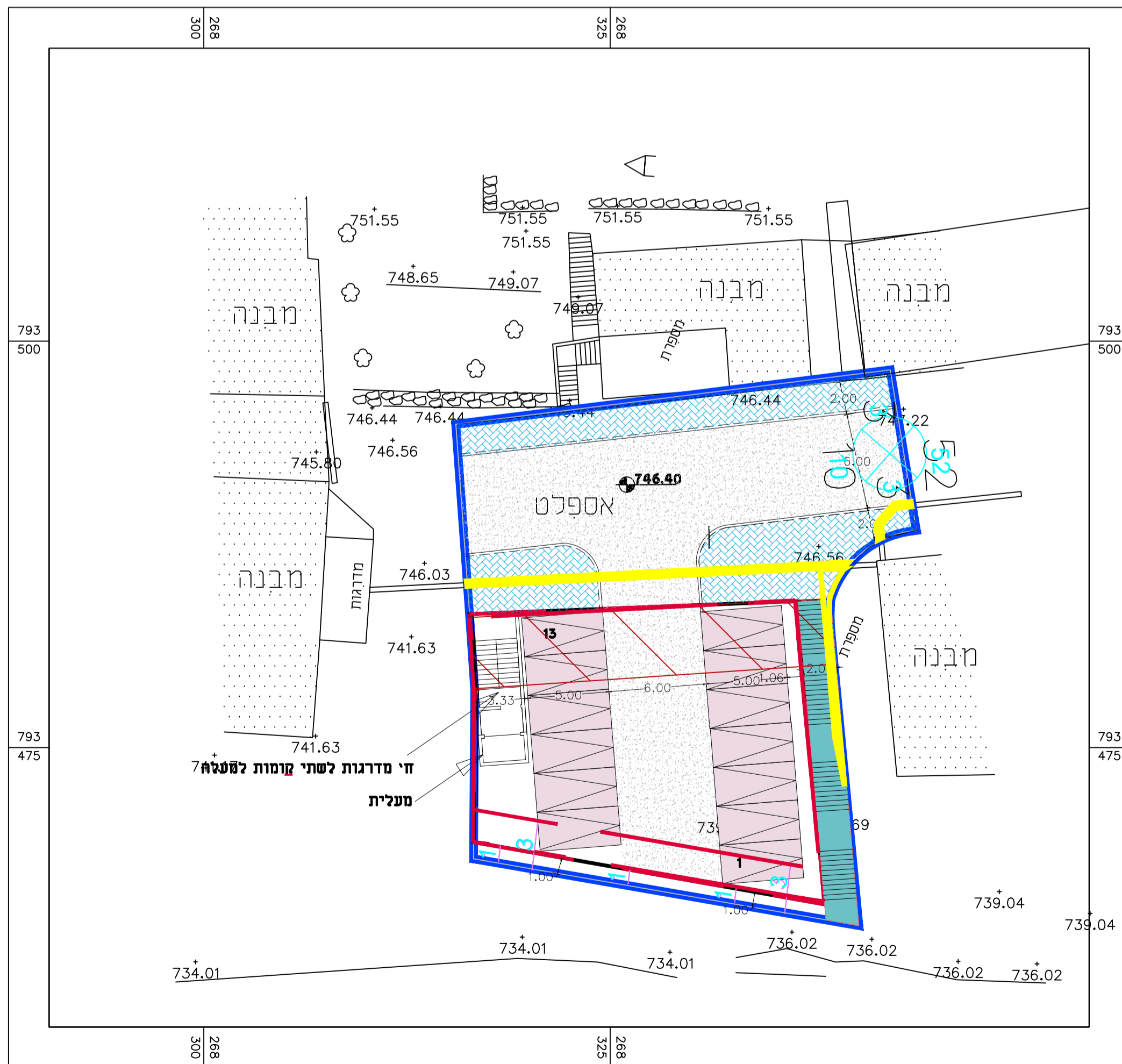
תכנית גג לשימוש חנייה
