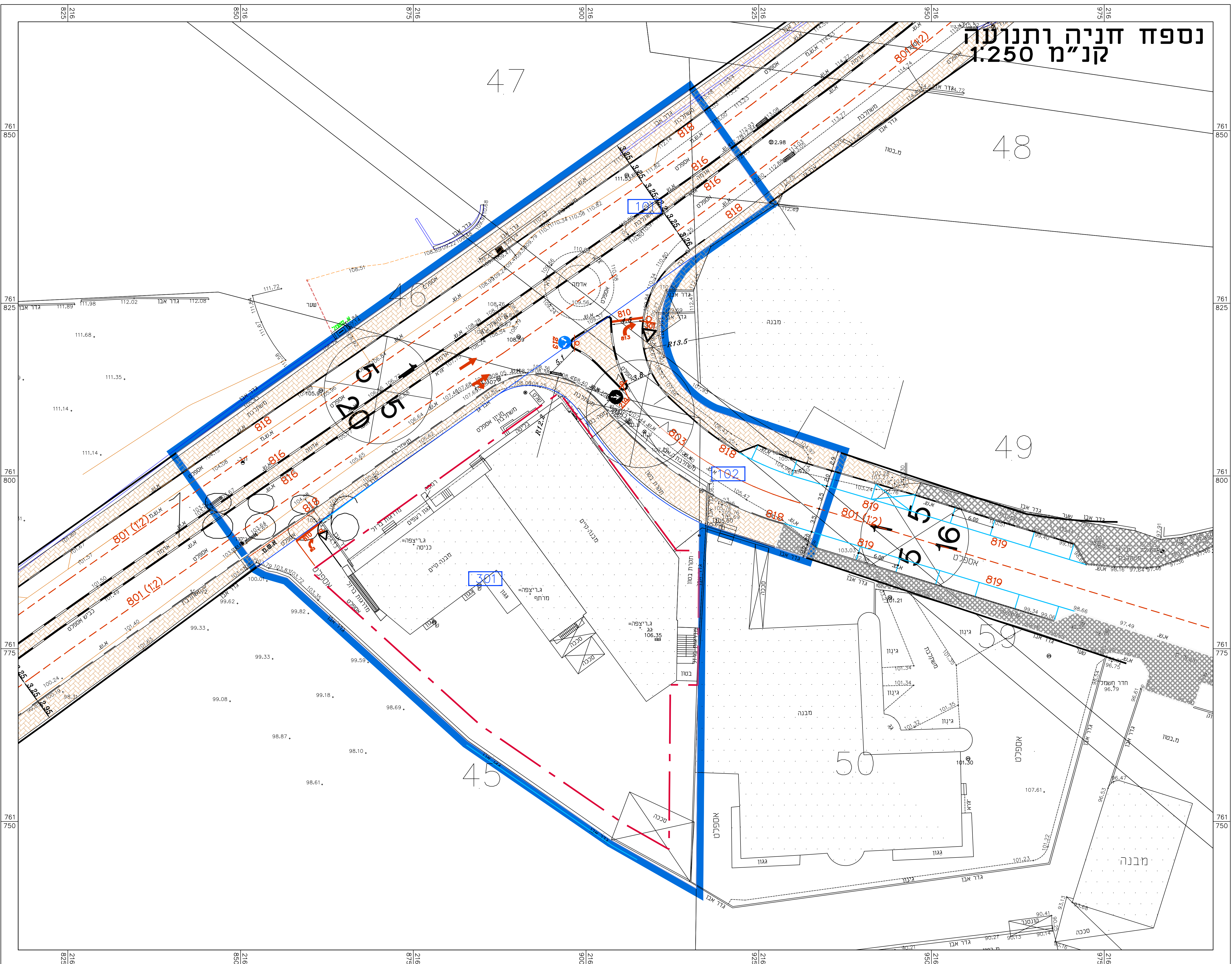
נספח חניה ותנועה קנ"מ 1:250
