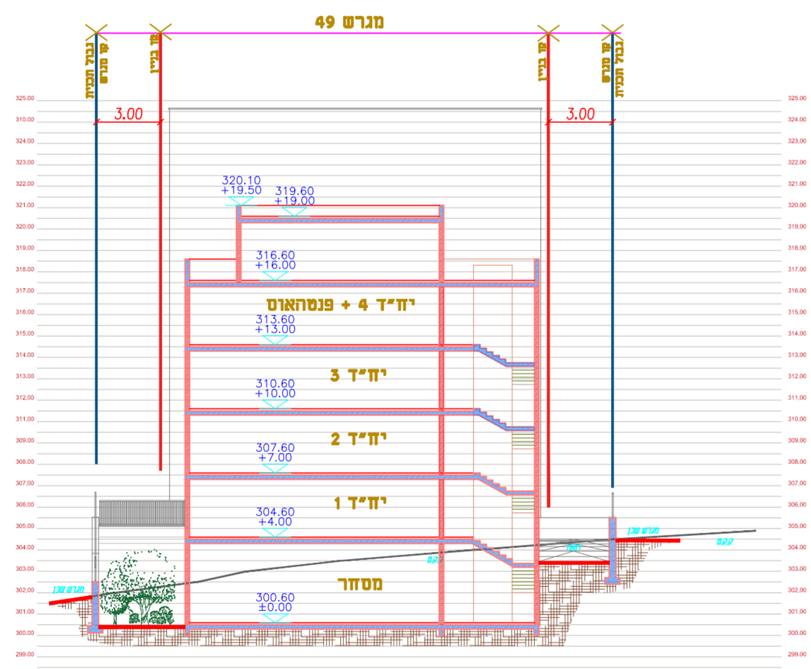
חתך 2-2 קנ"מ 1:250
