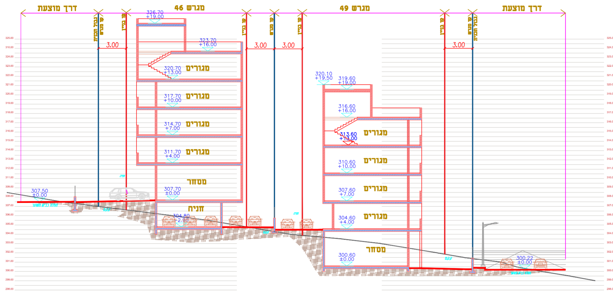
חתך 1-1 קנ"מ 1:250
