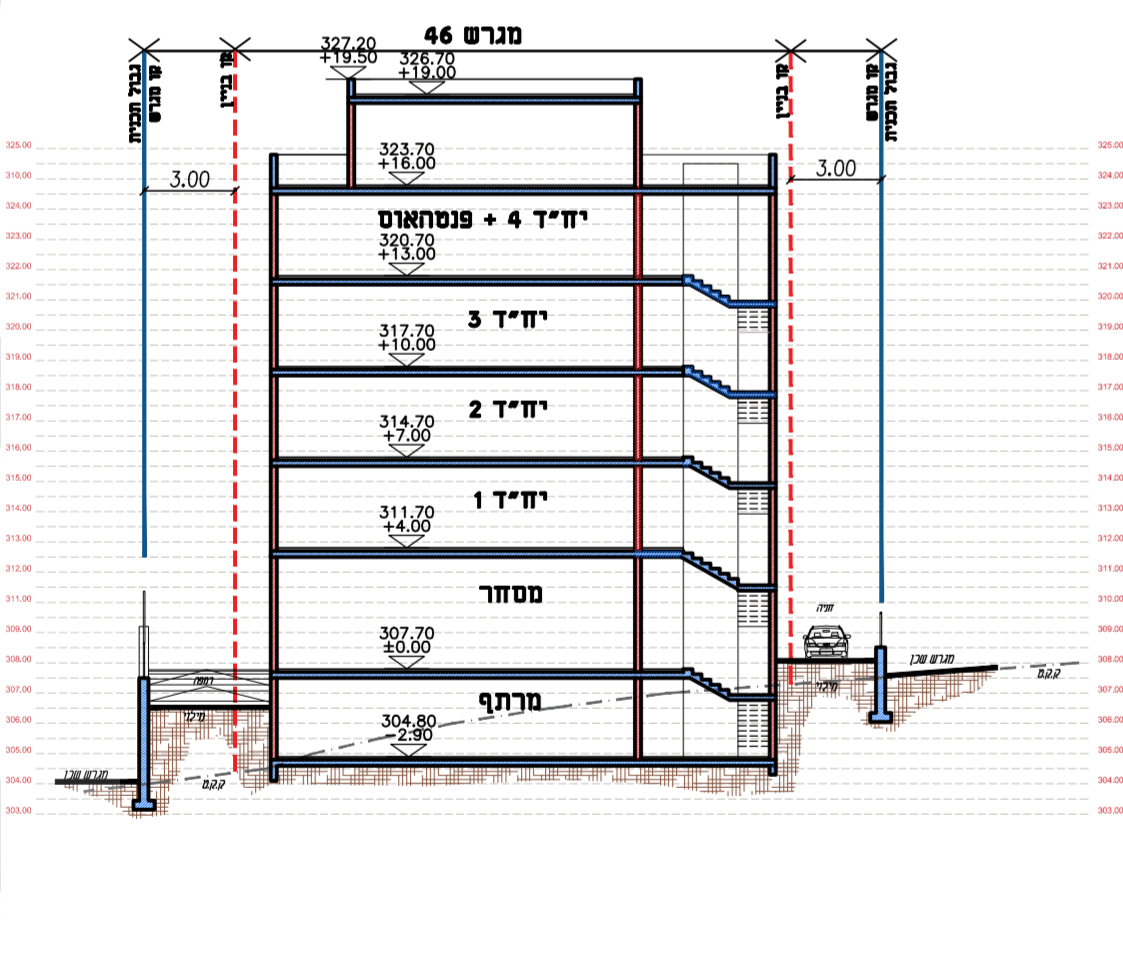
חתך 3-3 קנ"מ 1:250
