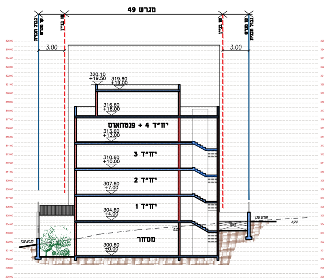
חתך 2-2 קנ"מ 1:250
