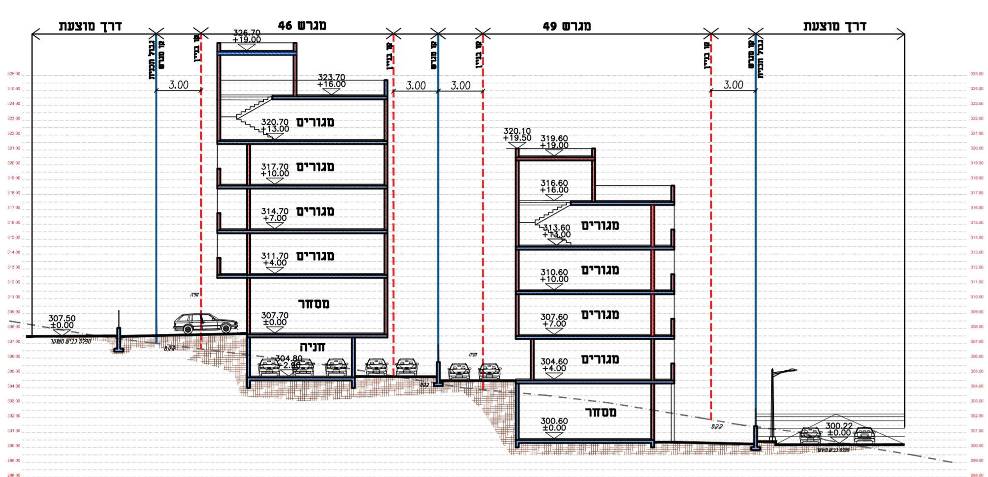
חתך 1-1 קנ"מ 1:250
