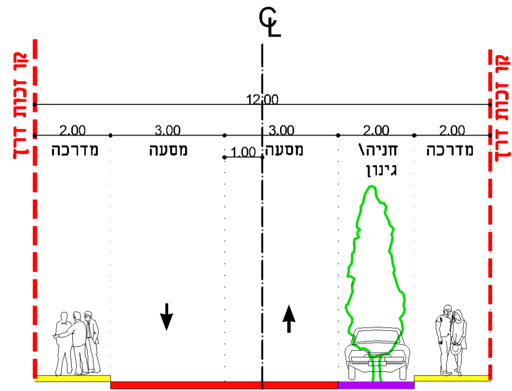
כביש ברוחב 12 מ' (כבישים 13, 11, 10, 3)
