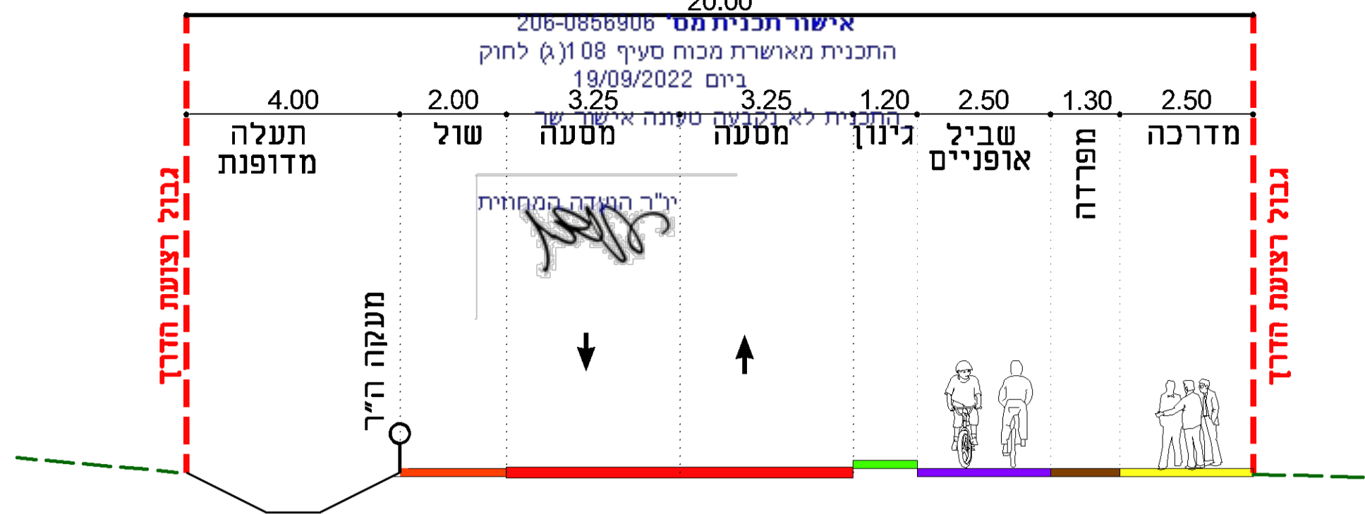
כביש ברוחב 20 מ' (כביש 1)
