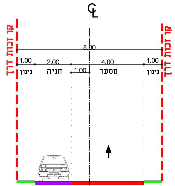
כביש ברוחב 8 מ' (רחוב משולב)
