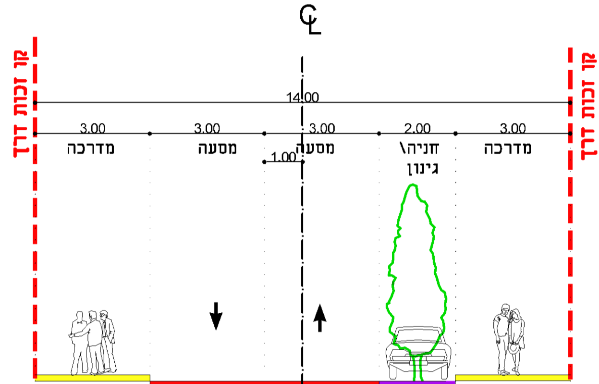
כביש ברוחב 14 מ' (כבישים 16, 9)
