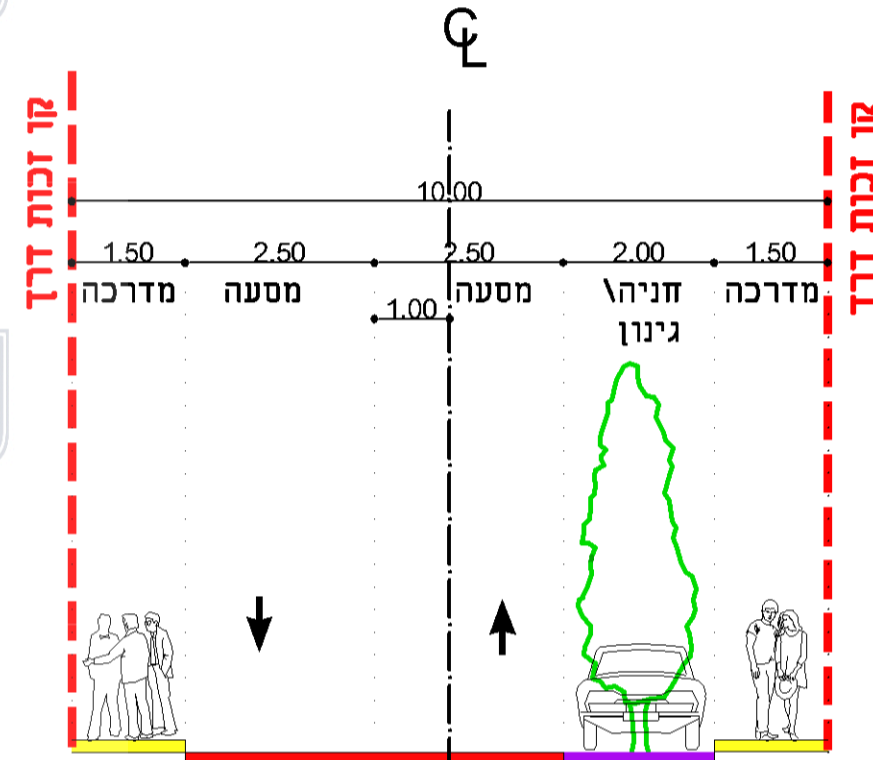
כביש ברוחב 10 מ' (כבישים 18, 15, 14)
