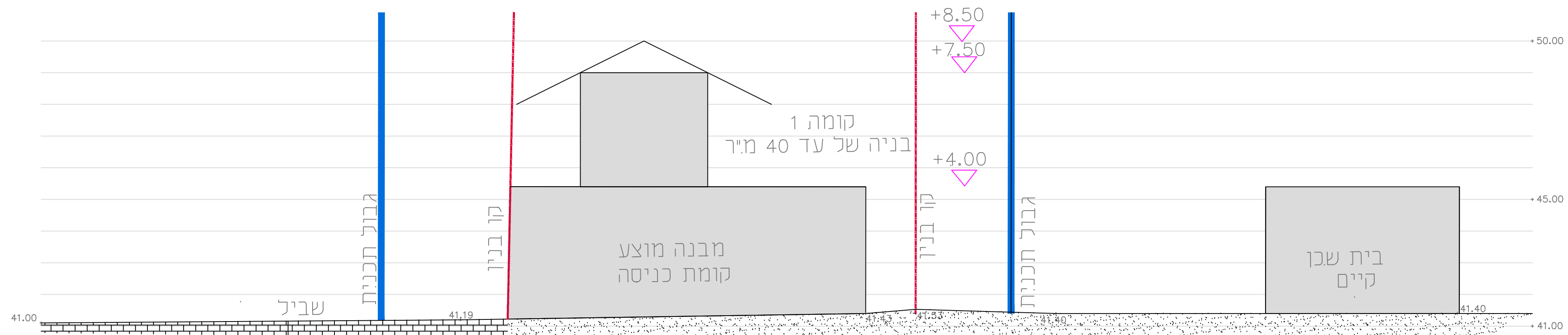
חתך א-א
