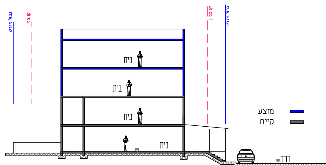
חיתוך בפי א-א קני"מ 1:100
