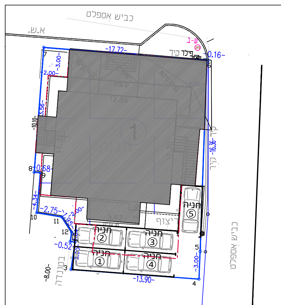
קומת קרקע קני"מ 1:100
