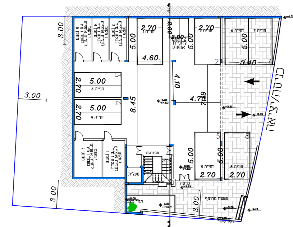
תוכנית חניון מס' 260
