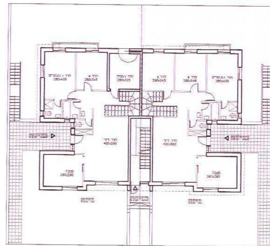
דירה 5 - שטח 2.97 מ"ר
