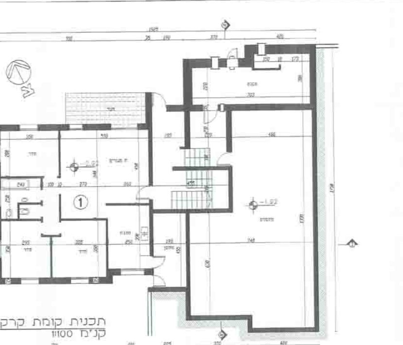
תכנית קומת קרקע קנ"מ 1:1000
