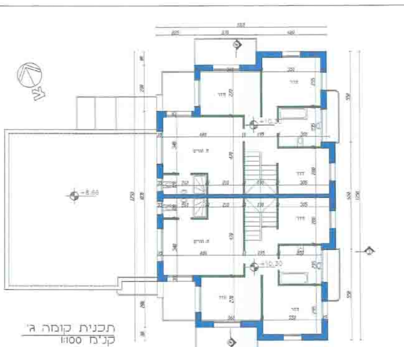
תכנית קומה ג' קנ"מ 1:1000
