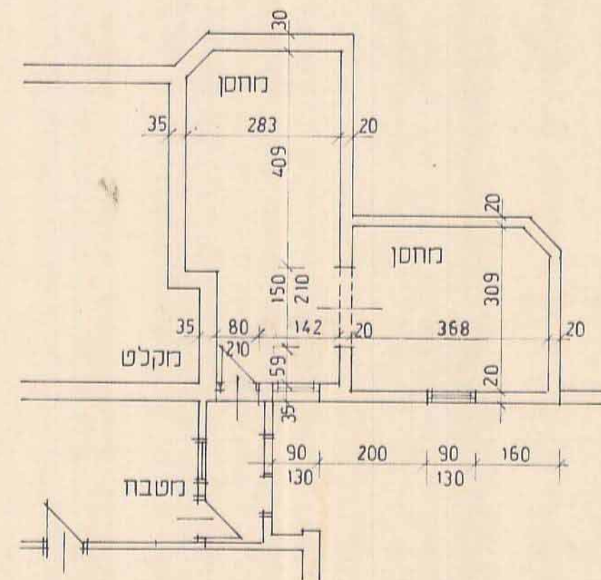
תכנית 1:100
