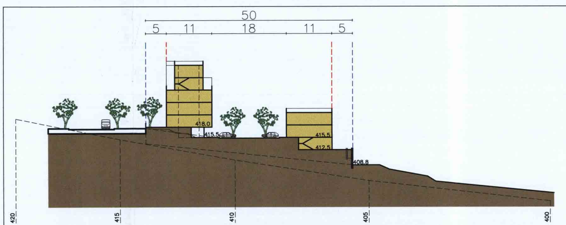
1:500 קנ"מ א-א חתך
