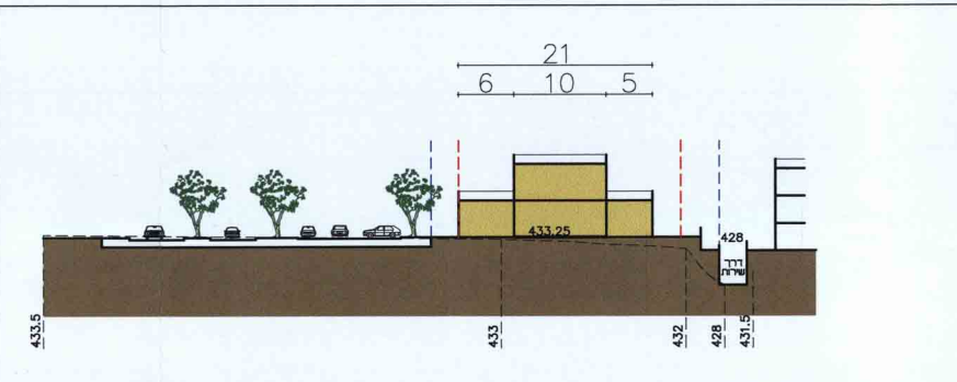
חתך ה-ה קנ"מ 1:500
