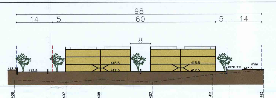
חתך ב-ב קנ"ח 1:500
