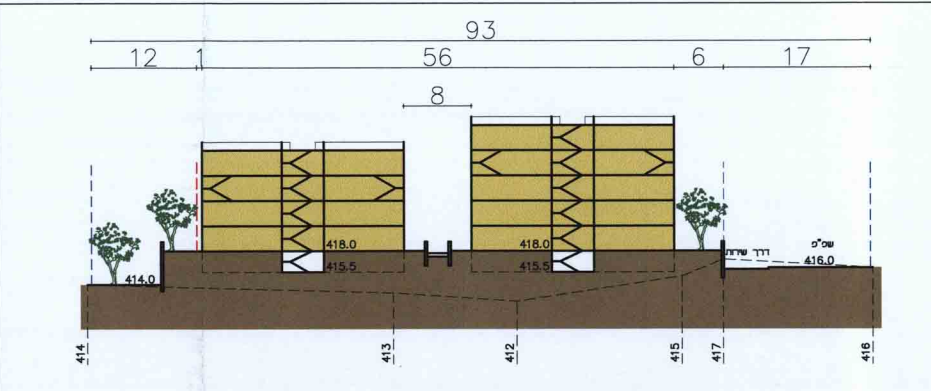
1:500 קנ"מ ג-ג חתך
