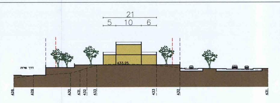
חתך ד-ד קנ"מ 1:500
