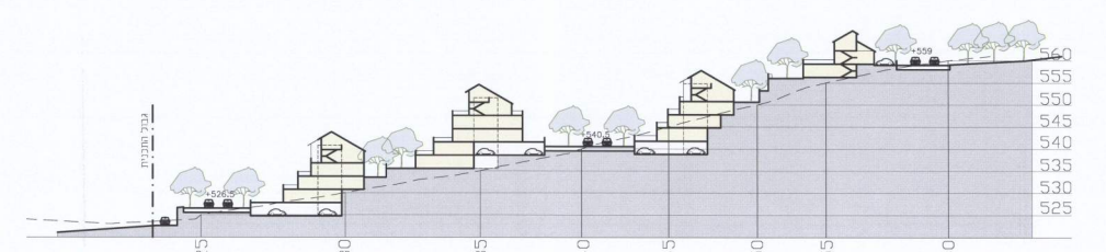
חתך 4-4
