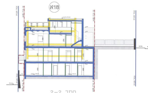
חתך 2-2 קנ"מ 1:100
