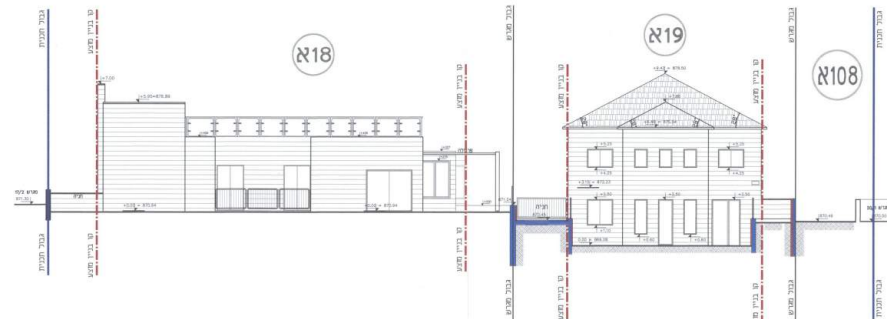
חזית דרומית קנ"מ 1:100
