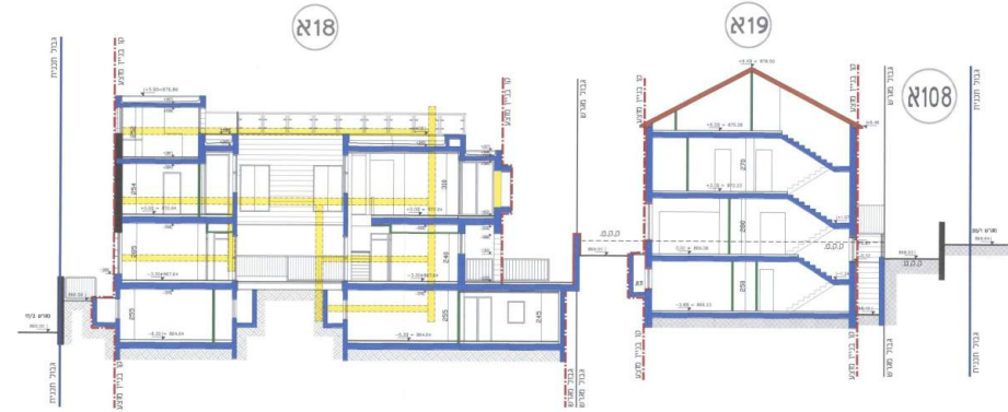
חתך 1-1 קנ"מ 1:100
