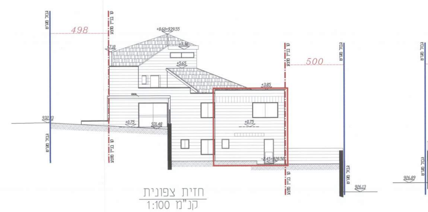
תכנית ב-ב ק"מ 1:100
