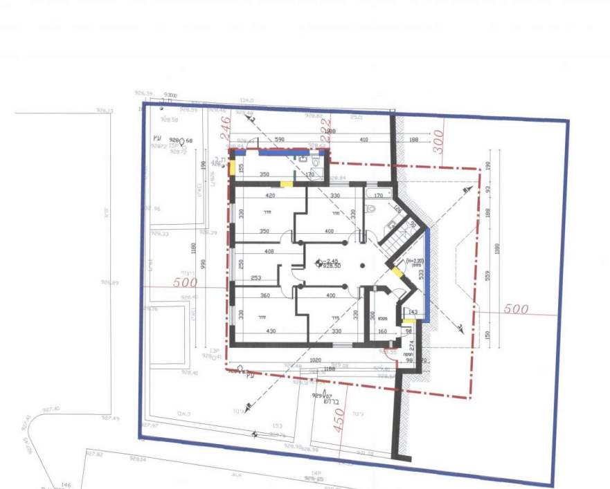
תכנית קומת התחנה ק"מ 1:100
