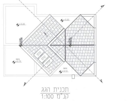
תכנית קומת א' ק"מ 1:100
