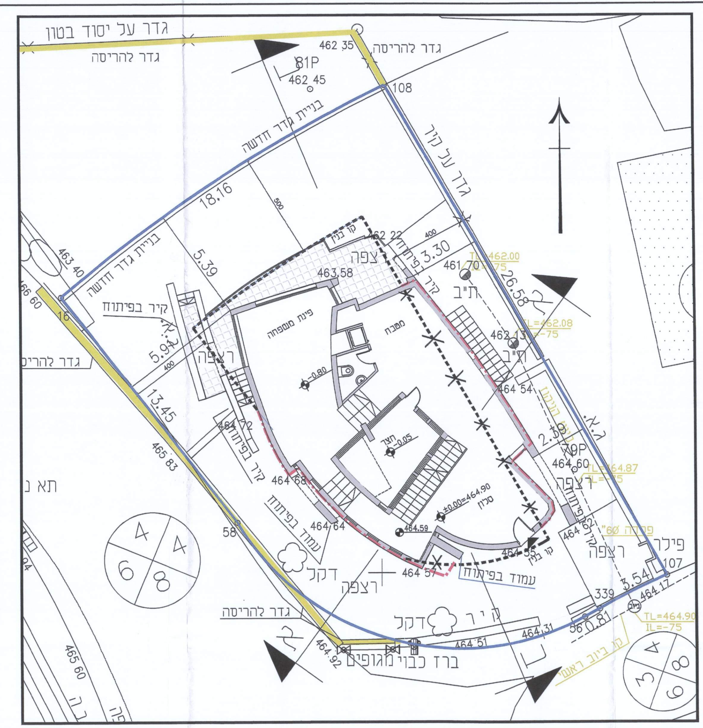
תכנית קומת מרתף ק"מ 1:100
