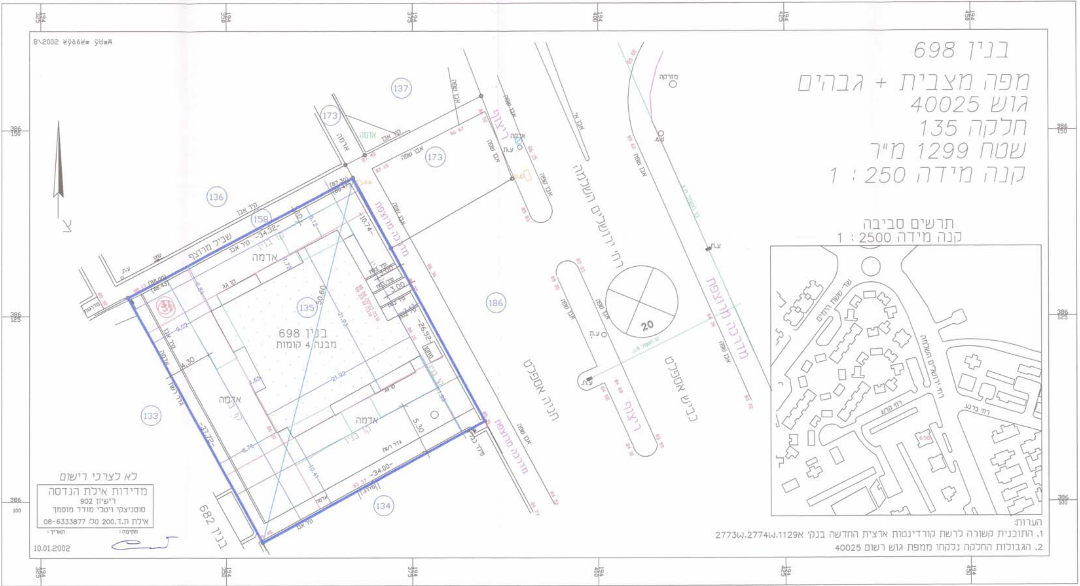
תרשים מיגרש קנ"מ. 1:250 מצב מוצע
