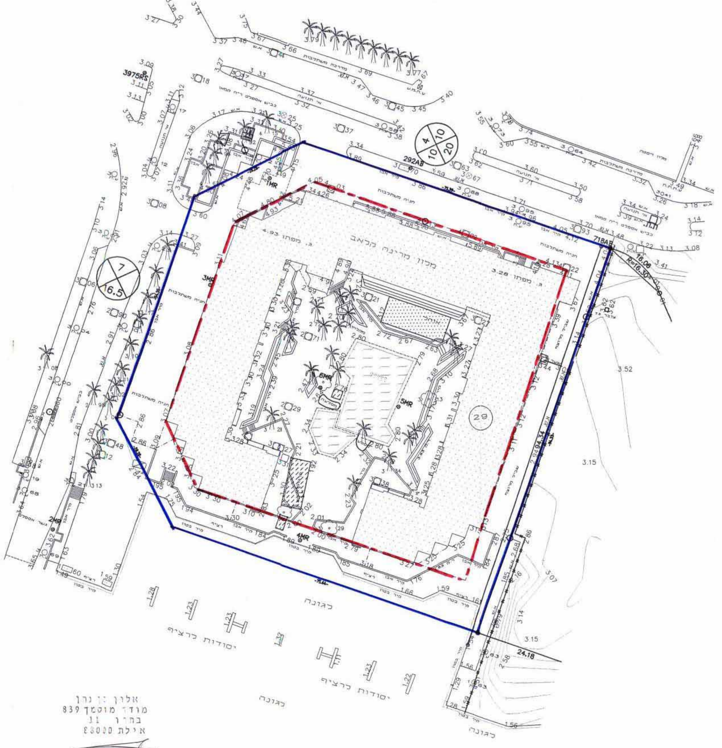
מצב קיים קנ"מ 1:500
