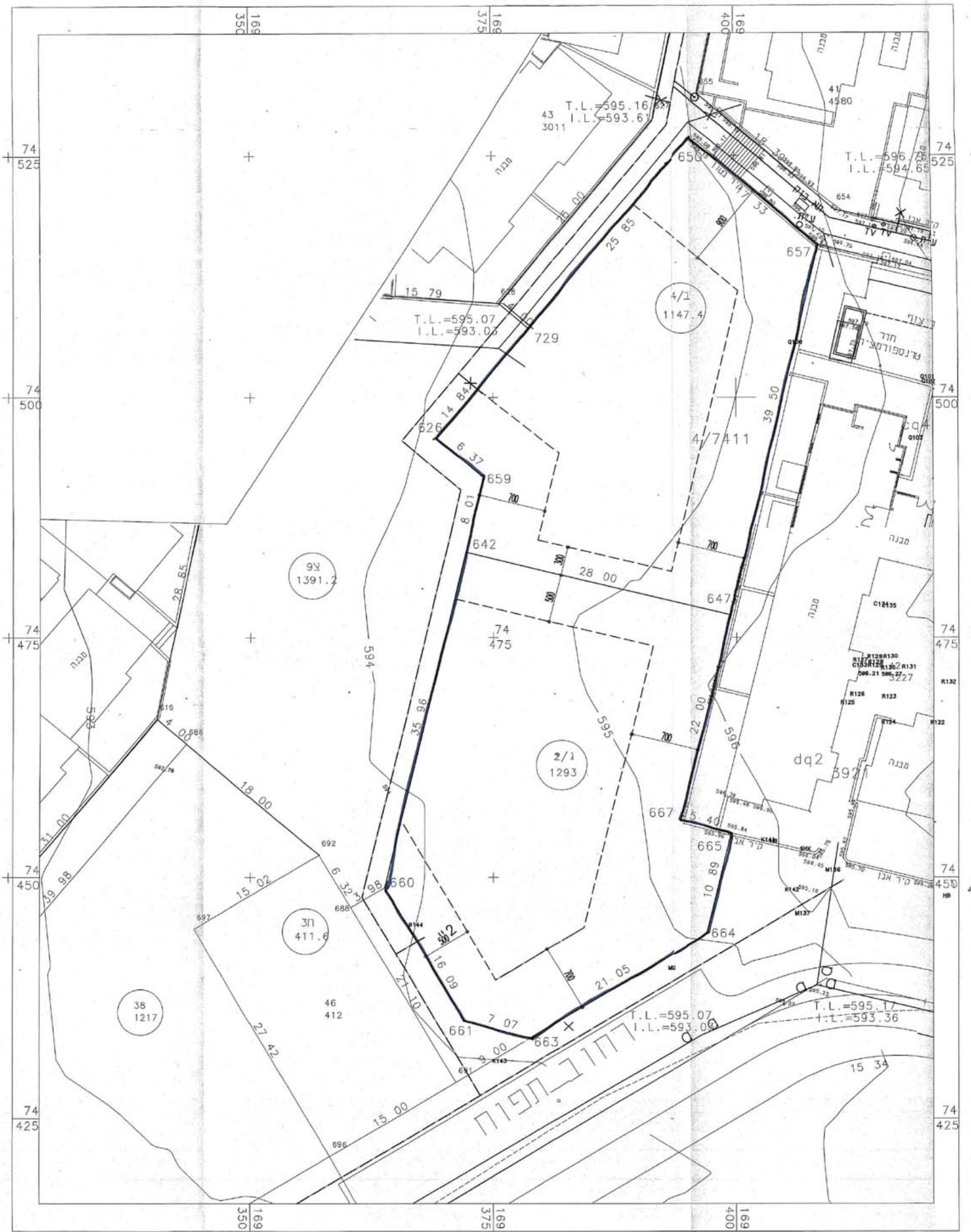
מצב קיים 1:250
