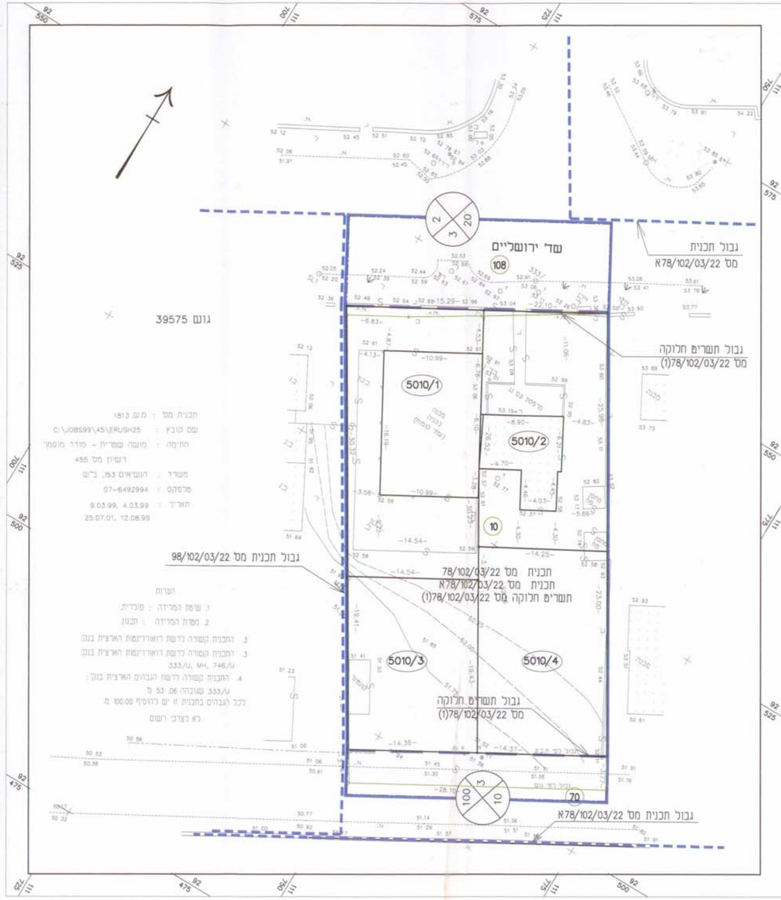
מצב קיים קני"מ 1:250
