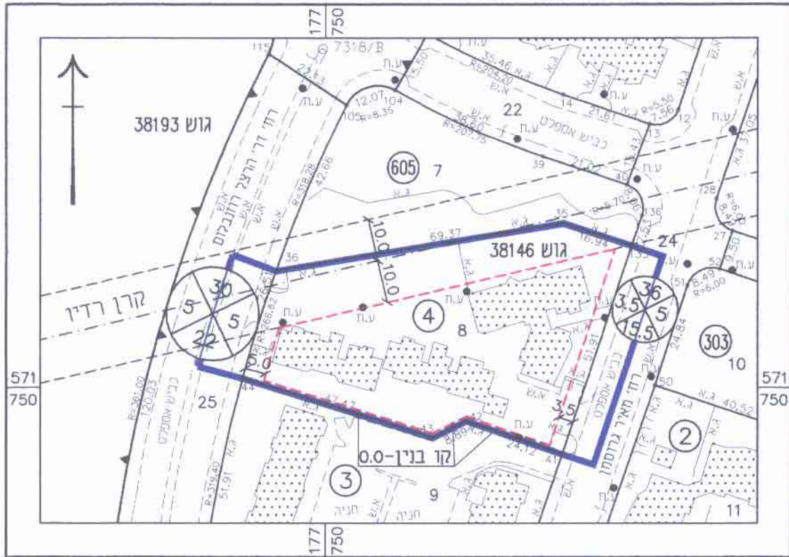
מצב קיים ומוצע קנ"מ 1:1250
