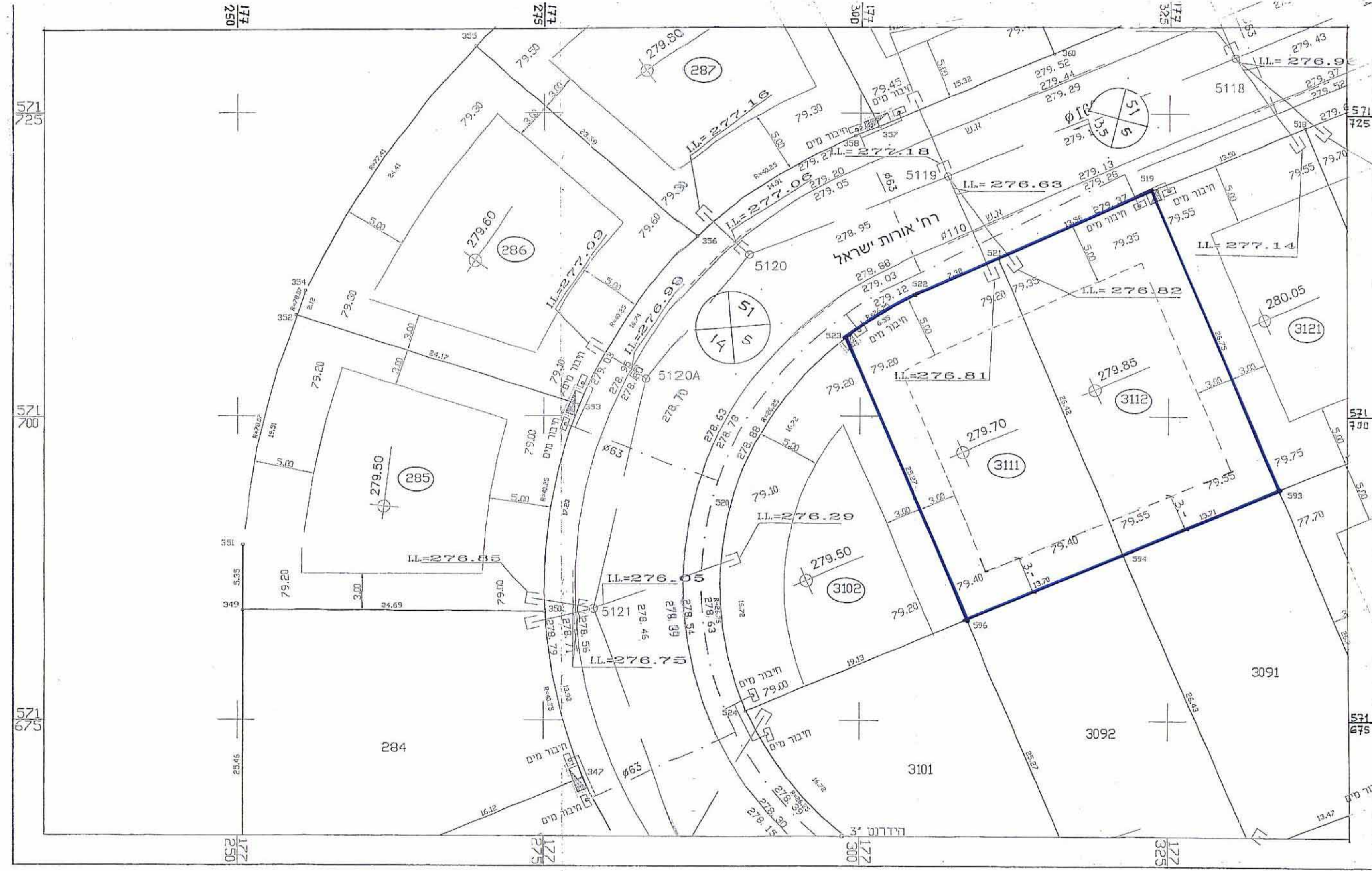
מצב מוצע 1:250
